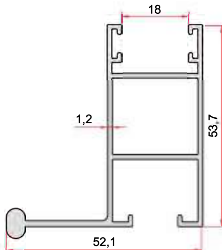
KOD-CODE TEORİK AĞIRLIK EP-1013 THEORETICAL WEIGHT 0,775 Kg/m
