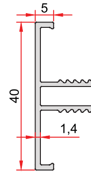
KOD-CODE TEORİK AĞIRLIK THEORETICAL WEIGHT EPAO-1042-14 0,286 Kg/m
