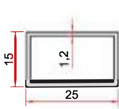
KOD-CODE TEORİK AĞIRLIK THEORETICAL WEIGHT EP-0046 0,243 Kg/m
