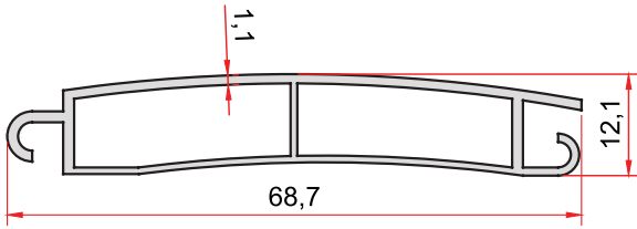
KOD-CODE TEORİK AĞIRLIK EP-2304 THEORETICAL WEIGHT 0,454 Kg/m
