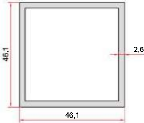
KOD-CODE TEORİK AĞIRLIK THEORETICAL WEIGHT EP-1965 1,220 Kg/m
