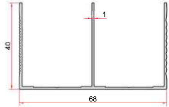
KOD-CODE TEORİK AĞIRLIK THEORETICAL WEIGHT EP-1458 0,543 Kg/m
