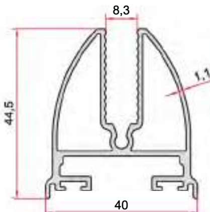
KOD-CODE TEORİK AĞIRLIK THEORETICAL WEIGHT EP-2718 0,781 Kg/m
