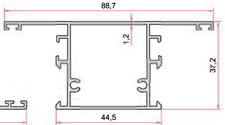
KOD-CODE TEORİK AĞIRLIK THEORETICAL WEIGHT EP-1132 0,859 Kg/m
