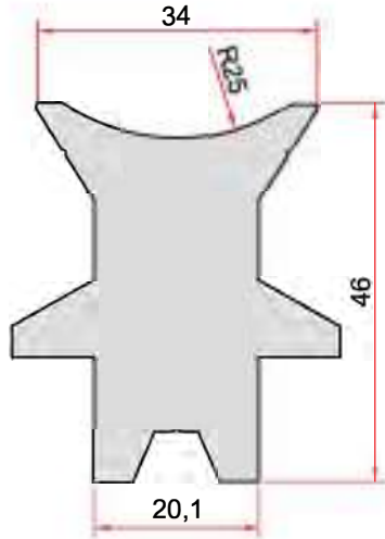
KOD-CODE TEORİK AĞIRLIK EP-1967 2,738 Kg/m
