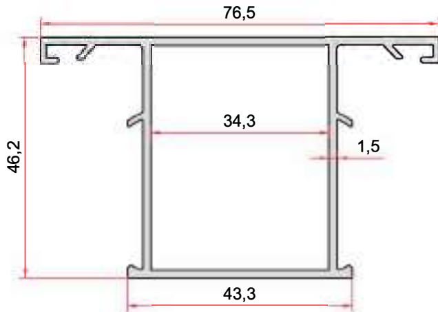
KOD-CODE TEORİK AĞIRLIK EP-0907 THEORETICAL WEIGHT 0,921 Kg/m
