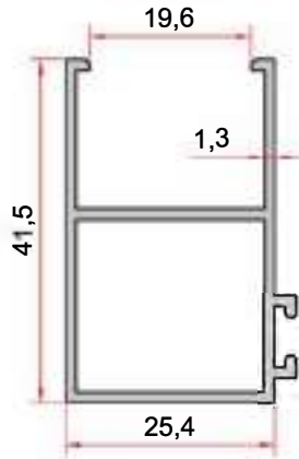
KOD-CODE TEORİK AĞIRLIK EP-1088 THEORETICAL WEIGHT 0,489 Kg/m
