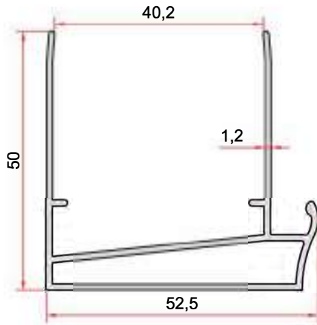
KOD-CODE TEORİK AĞIRLIK THEORETICAL WEIGHT EP-2664 0,680 Kg/m
