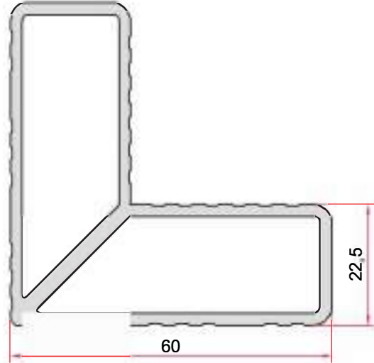
KOD-CODE TEORİK AĞIRLIK EPKT-225-00 THEORETICAL WEIGHT 1,508 Kg/m
