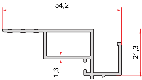
KOD-CODE TEORİK AĞIRLIK THEORETICAL WEIGHT EPAO-1022-13 0,453 Kg/m
