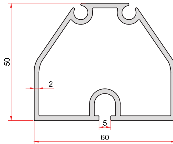
KOD-CODE TEORİK AĞIRLIK EP-0098 THEORETICAL WEIGHT 1,223 Kg/m
