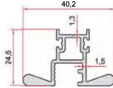
KOD-CODE TEORİK AĞIRLIK THEORETICAL WEIGHT EP-2723 0,545 Kg/m
