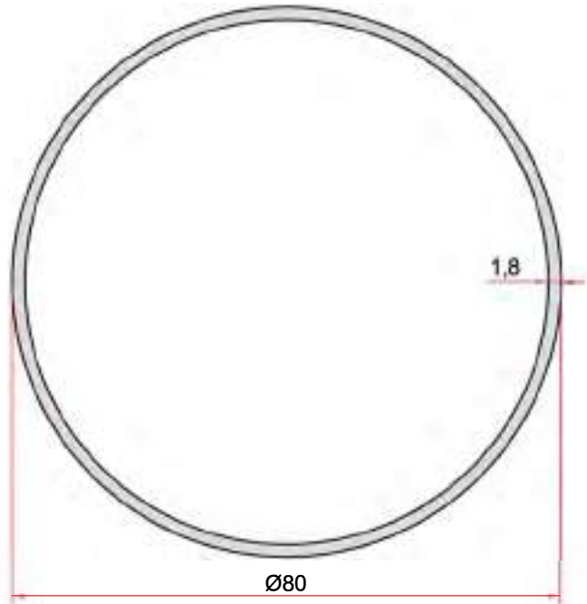
KOD-CODE TEORİK AĞIRLIK EP-1936 THEORETICAL WEIGHT 1,193 Kg/m
