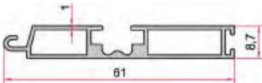
KOD-CODE TEORİK AĞIRLIK THEORETICAL WEIGHT EP-1093 0,437 Kg/m
