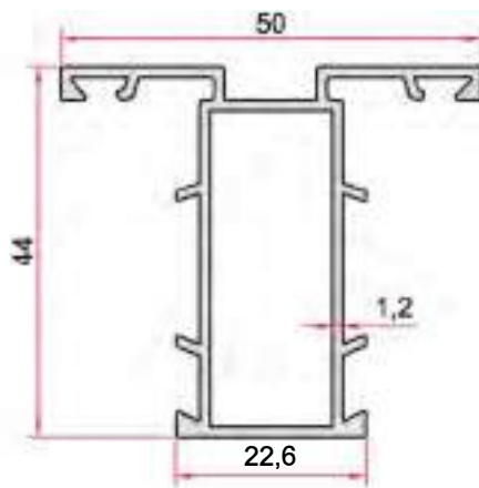
KOD-CODE TEORİK AĞIRLIK EP-1083 0,626 Kg/m
