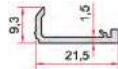
KOD-CODE TEORİK AĞIRLIK THEORETICAL WEIGHT EPİS-302-15 0,130 Kg/m
