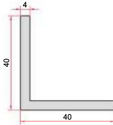
KOD-CODE TEORİK AĞIRLIK THEORETICAL WEIGHT EP-0139 0,820 Kg/m
