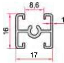
KOD-CODE TEORİK AĞIRLIK THEORETICAL WEIGHT EP-1398 0,200 Kg/m
