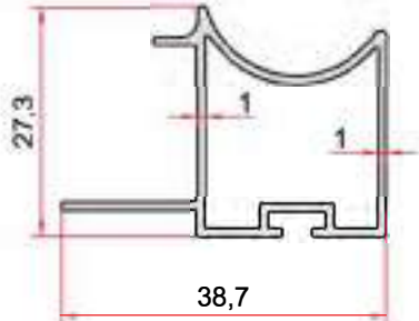
KOD-CODE TEORİK AĞIRLIK THEORETICAL WEIGHT EP-1510 0,345 Kg/m
