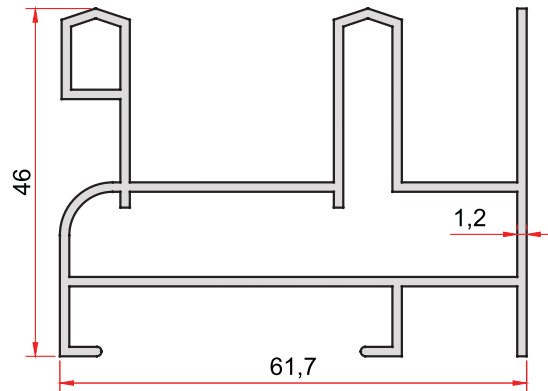
KOD-CODE TEORİK AĞIRLIK EP-803 THEORETICAL WEIGHT 0,999 Kg/m
