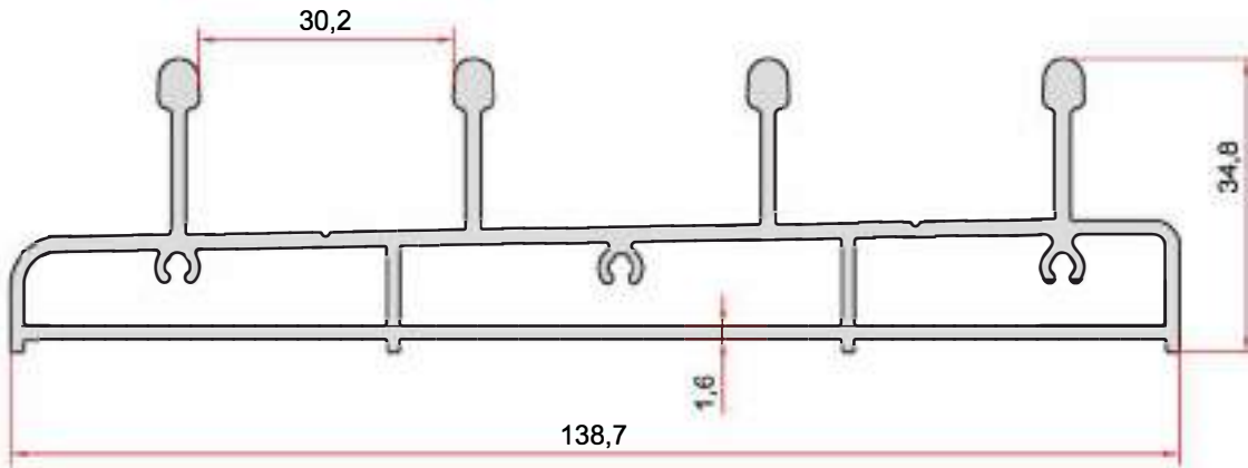
KOD-CODE EP-2670 TEORİK AĞIRLIK THEORETICAL WEIGHT 2,107 Kg/m
