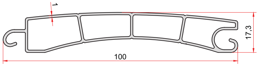
KOD-CODE TEORİK AĞIRLIK EP-2311 THEORETICAL WEIGHT 0,748 Kg/m
