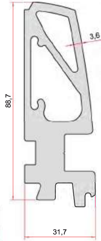
KOD-CODE TEORİK AĞIRLIK THEORETICAL WEIGHT EP-2276 3,591 Kg/m
