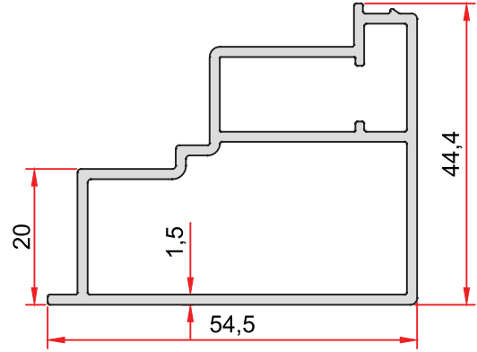
KOD-CODE TEORİK AĞIRLIK EPAO-1025-15 THEORETICAL WEIGHT 0,871 Kg/m
