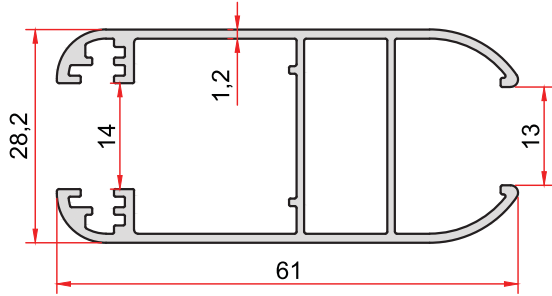
KOD-CODE TEORİK AĞIRLIK EP-784 THEORETICAL WEIGHT 0,685 Kg/m
