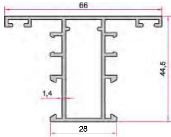
KOD-CODE TEORİK AĞIRLIK EP-1084 0,886 Kg/m
