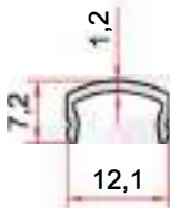
KOD-CODE TEORİK AĞIRLIK THEORETICAL WEIGHT EP-1956 0,064 Kg/m
