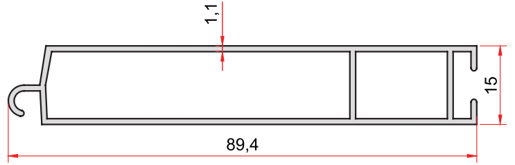
KOD-CODE TEORİK AĞIRLIK EP-2302 THEORETICAL WEIGHT 0,659 Kg/m
