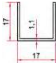
KOD-CODE TEORİK AĞIRLIK THEORETICAL WEIGHT EP-0083 0,146 Kg/m
