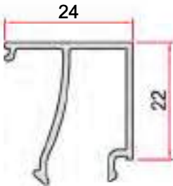
KOD-CODE TEORİK AĞIRLIK THEORETICAL WEIGHT EPCC-1240-13 0,285 Kg/m
