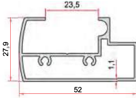
KOD-CODE TEORİK AĞIRLIK THEORETICAL WEIGHT EP-1754 0,596 Kg/m
