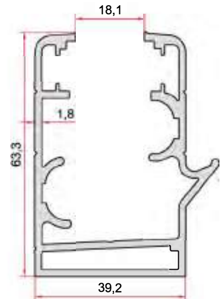
KOD-CODE TEORİK AĞIRLIK THEORETICAL WEIGHT EP-2653 1,393 Kg/m
