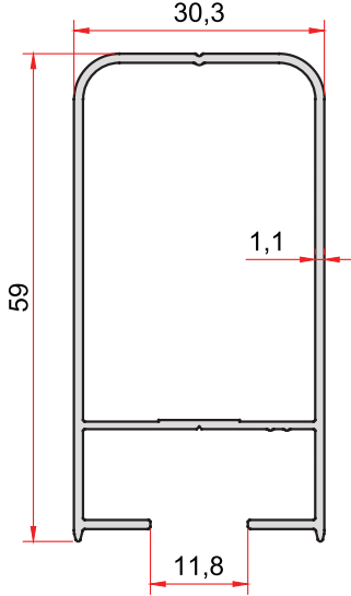
KOD-CODE TEORİK AĞIRLIK EP-769 THEORETICAL WEIGHT 0,543 Kg/m
