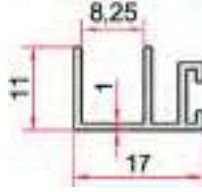
KOD-CODE TEORİK AĞIRLIK THEORETICAL WEIGHT EP-2625 0,135 Kg/m
