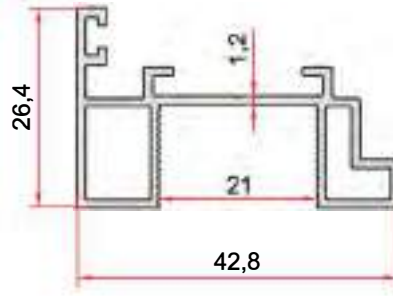
KOD-CODE TEORİK AĞIRLIK THEORETICAL WEIGHT EP-2733 0,443 Kg/m
