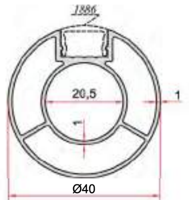
KOD-CODE TEORİK AĞIRLIK THEORETICAL WEIGHT EP-2000 0,607 Kg/m
