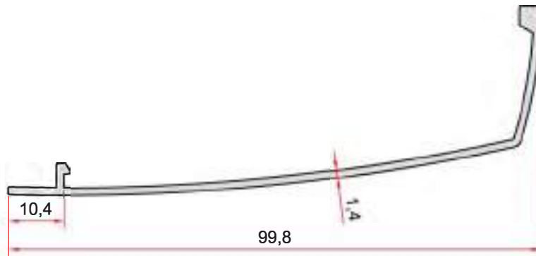
KOD-CODE TEORİK AĞIRLIK THEORETICAL WEIGHT EP-2275 0,510 Kg/m
