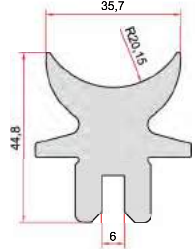
KOD-CODE TEORİK AĞIRLIK EP-1866 2,400 Kg/m
