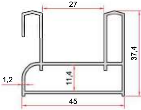
KOD-CODE TEORİK AĞIRLIK THEORETICAL WEIGHT EP-1123 0,664 Kg/m
