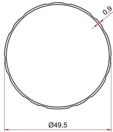
KOD-CODE TEORİK AĞIRLIK THEORETICAL WEIGHT EP-4021 0,356 Kg/m
