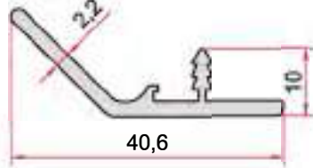
KOD-CODE TEORİK AĞIRLIK THEORETICAL WEIGHT EP-1474 0,324 Kg/m
