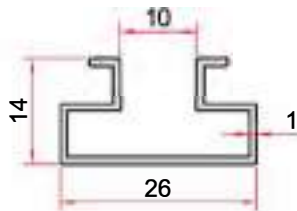
KOD-CODE TEORİK AĞIRLIK THEORETICAL WEIGHT EP-1451 0,194 Kg/m
