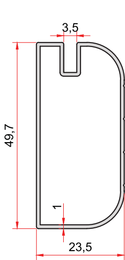
KOD-CODE TEORİK AĞIRLIK EP-877 THEORETICAL WEIGHT 0,402 Kg/m
