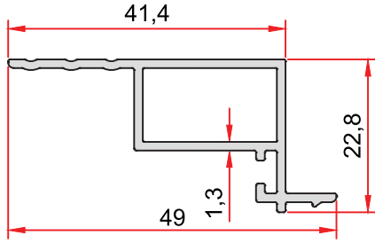
KOD-CODE TEORİK AĞIRLIK THEORETICAL WEIGHT EPAO-1021-13 0,384 Kg/m
