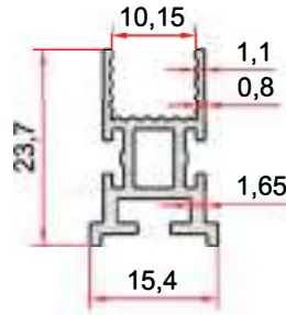
KOD-CODE TEORİK AĞIRLIK THEORETICAL WEIGHT EP-2722 0,267 Kg/m
