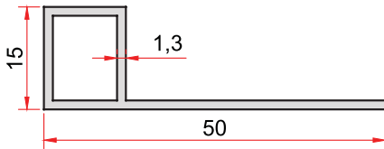
KOD-CODE TEORİK AĞIRLIK EP-4020 THEORETICAL WEIGHT 0,302 Kg/m
