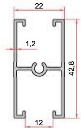
KOD-CODE TEORİK AĞIRLIK THEORETICAL WEIGHT EP-1082 0,437 Kg/m
