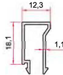
KOD-CODE TEORİK AĞIRLIK EP5S-302-11 THEORETICAL WEIGHT 0,176 Kg/m
