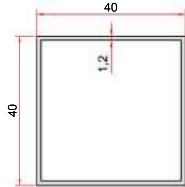
KOD-CODE TEORİK AĞIRLIK THEORETICAL WEIGHT EP-0056 0,502 Kg/m
