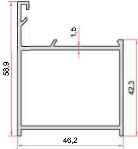
KOD-CODE TEORİK AĞIRLIK EP-0905 THEORETICAL WEIGHT 0,801 Kg/m
