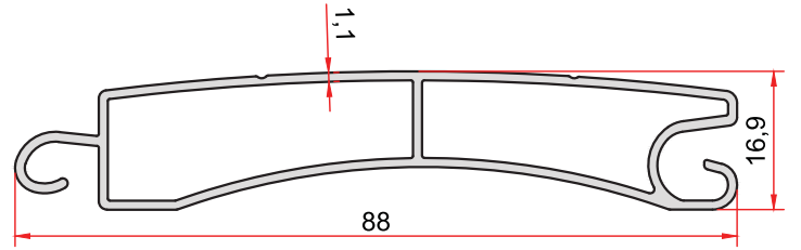
KOD-CODE TEORİK AĞIRLIK EP-2315 THEORETICAL WEIGHT 0,667 Kg/m
