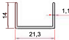
KOD-CODE TEORİK AĞIRLIK THEORETICAL WEIGHT EP-1388 0,140 Kg/m
