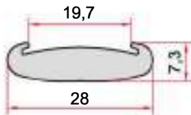
KOD-CODE TEORİK AĞIRLIK EP-1454 THEORETICAL WEIGHT 0,429 Kg/m
