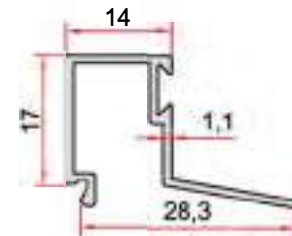
KOD-CODE TEORİK AĞIRLIK EP-0835 THEORETICAL WEIGHT 0,205 Kg/m
