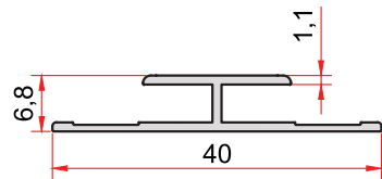
KOD-CODE TEORİK AĞIRLIK EP-1061 THEORETICAL WEIGHT 0,173 Kg/m
