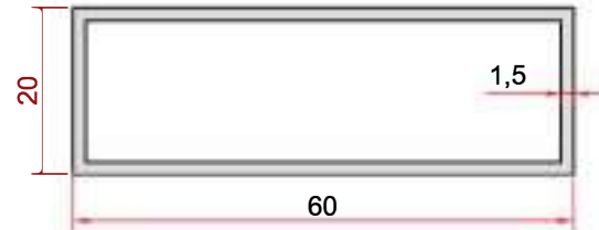
KOD-CODE TEORİK AĞIRLIK THEORETICAL WEIGHT EP-0111 0,623 Kg/m
