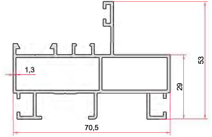
KOD-CODE TEORİK AĞIRLIK THEORETICAL WEIGHT EP-7034 1,085 Kg/m
