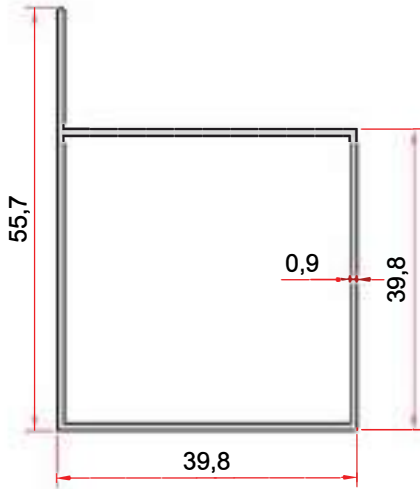
KOD-CODE TEORİK AĞIRLIK THEORETICAL WEIGHT EP-1435 0,416 Kg/m
