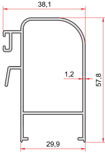
KOD-CODE TEORİK AĞIRLIK THEORETICAL WEIGHT EP- 874 0,656 Kg/m
