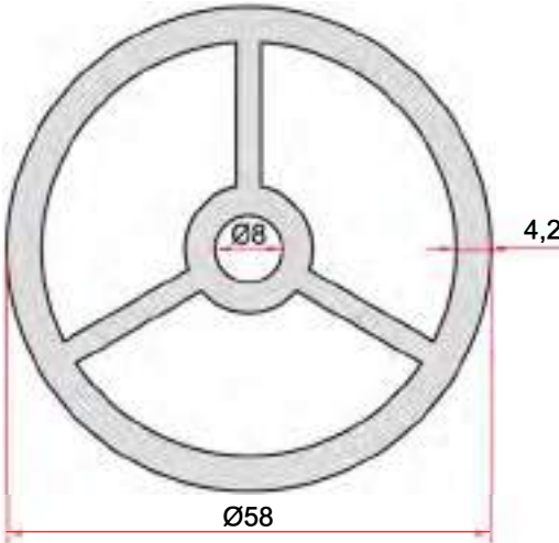
KOD-CODE TEORİK AĞIRLIK EP-1964 2,692 Kg/m THEORETICAL WEIGHT
