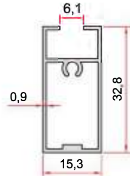
KOD-CODE TEORİK AĞIRLIK THEORETICAL WEIGHT EP-1759 0,278 Kg/m
