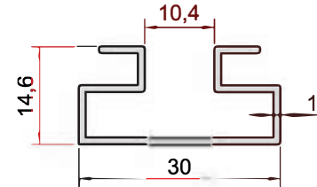
KOD-CODE TEORİK AĞIRLIK THEORETICAL WEIGHT EP-1389 0,232 Kg/m
