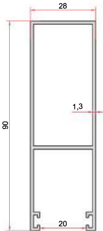
KOD-CODE TEORİK AĞIRLIK EP-7009 THEORETICAL WEIGHT 0,861 Kg/m
