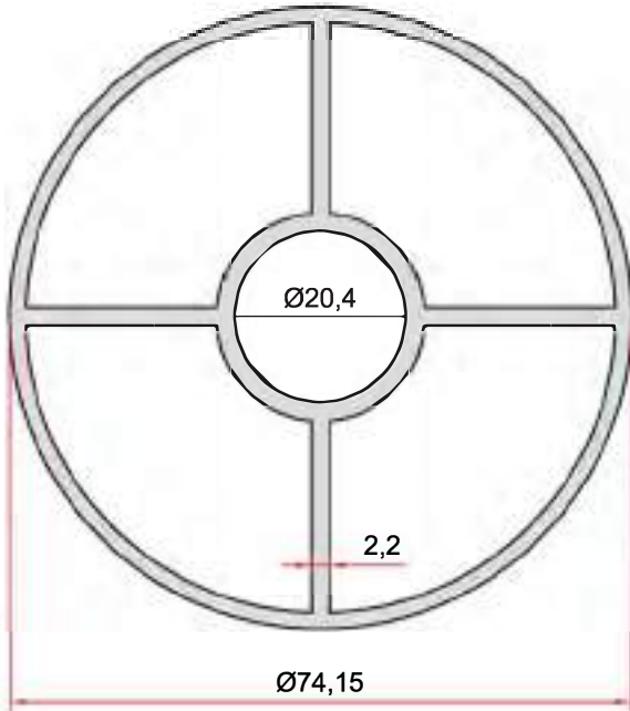
KOD-CODE TEORİK AĞIRLIK EP-1958 THEORETICAL WEIGHT 2,127 Kg/m
