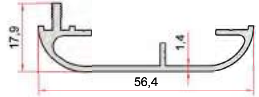
KOD-CODE TEORİK AĞIRLIK THEORETICAL WEIGHT EP-1106 0,421 Kg/m
