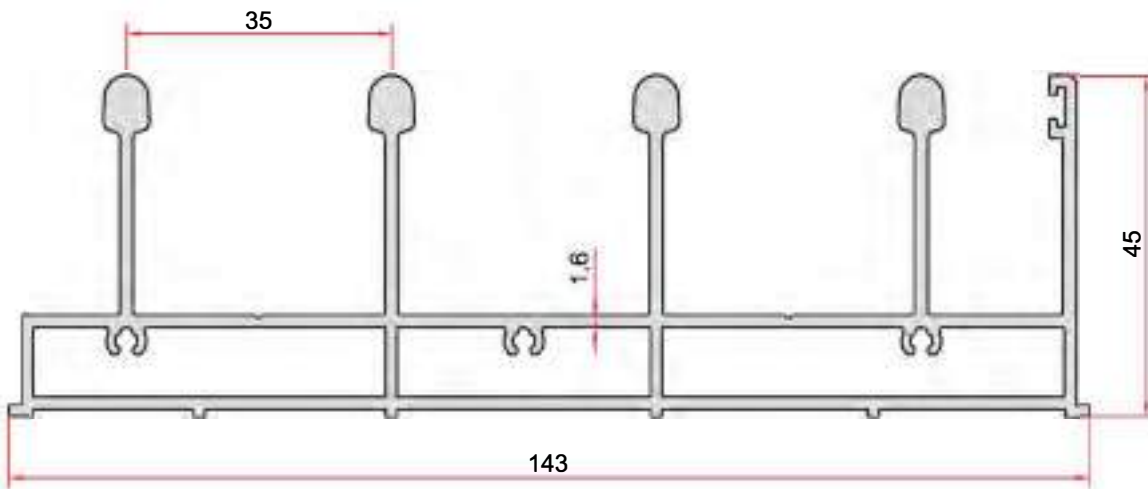
KOD-CODE EP-2669 TEORİK AĞIRLIK THEORETICAL WEIGHT 2,538 Kg/m
