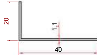
KOD-CODE TEORİK AĞIRLIK EP-0017 THEORETICAL WEIGHT 0,176 Kg/m
