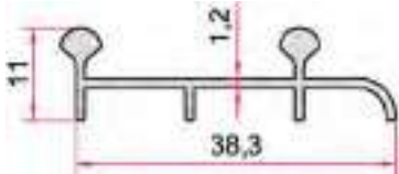
KOD-CODE TEORİK AĞIRLIK THEORETICAL WEIGHT EP-1402 0,246 Kg/m
