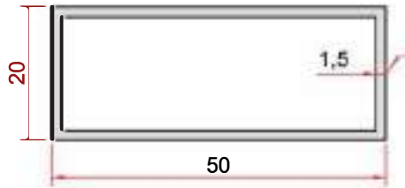
KOD-CODE TEORİK AĞIRLIK THEORETICAL WEIGHT EP-0115 0,542 Kg/m
