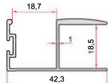
KOD-CODE TEORİK AĞIRLIK THEORETICAL WEIGHT EP-1466 0,378 Kg/m
