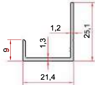
KOD-CODE TEORİK AĞIRLIK THEORETICAL WEIGHT EP-1377 0,178 Kg/m
