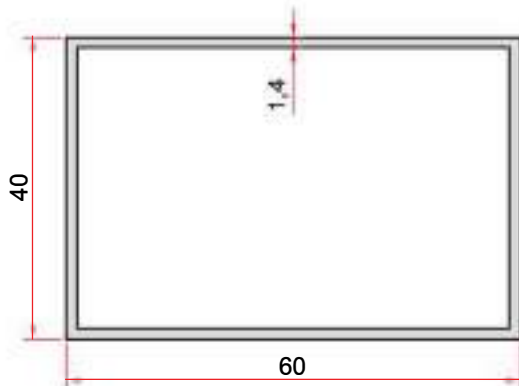
KOD-CODE TEORİK AĞIRLIK THEORETICAL WEIGHT EP-0024 0,734 Kg/m
