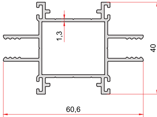
KOD-CODE TEORİK AĞIRLIK THEORETICAL WEIGHT EPAO-1011-13 0,805 Kg/m
