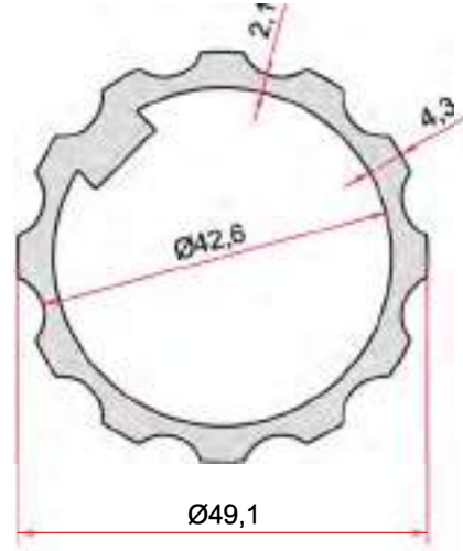
KOD-CODE TEORİK AĞIRLIK THEORETICAL WEIGHT EP-1968 1,350 Kg/m
