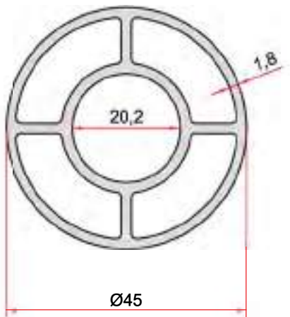
KOD-CODE TEORİK AĞIRLIK EP-1859 1,231 Kg/m THEORETICAL WEIGHT
