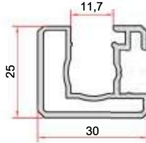
KOD-CODE TEORİK AĞIRLIK THEORETICAL WEIGHT EP-1908 0,508 Kg/m
