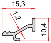
KOD-CODE TEORİK AĞIRLIK THEORETICAL WEIGHT EPAO-1031-12 0,084 Kg/m
