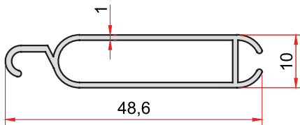
KOD-CODE TEORİK AĞIRLIK EP-2305 THEORETICAL WEIGHT 0,297 Kg/m
