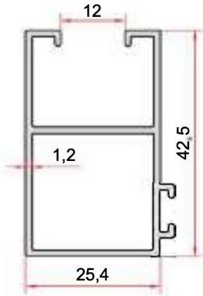
KOD-CODE TEORİK AĞIRLIK EP-1011 THEORETICAL WEIGHT 0,495 Kg/m
