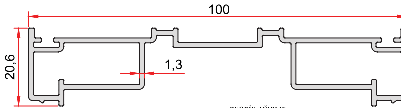
KOD-CODE TEORİK AĞIRLIK THEORETICAL WEIGHT EPAO-1012-13 0,874 Kg/m
