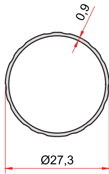
KOD-CODE TEORİK AĞIRLIK THEORETICAL WEIGHT EP-4022 0,189 Kg/m
