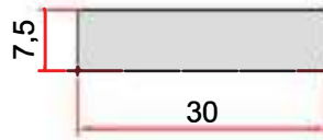
KOD-CODE TEORİK AĞIRLIK EP-1407 THEORETICAL WEIGHT 0,607 Kg/m
