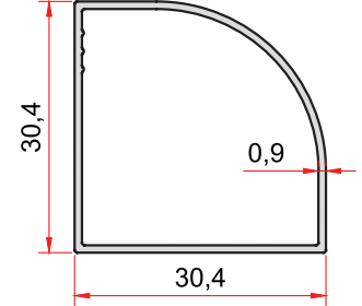
KOD-CODE TEORİK AĞIRLIK EP-774 THEORETICAL WEIGHT 0,267 Kg/m
