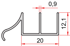
KOD-CODE TEORİK AĞIRLIK EP-777 THEORETICAL WEIGHT 0,176 Kg/m
