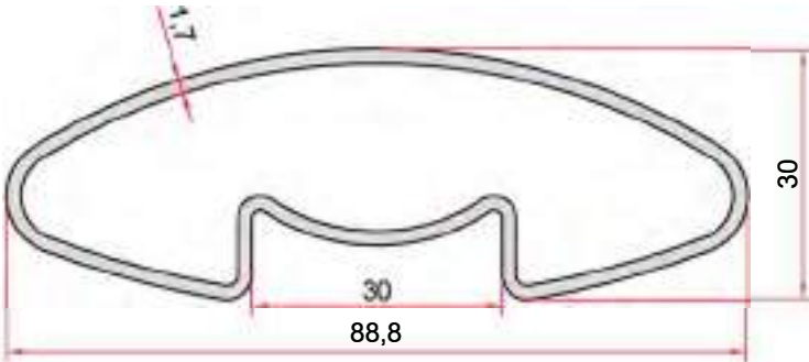
KOD-CODE TEORİK AĞIRLIK THEORETICAL WEIGHT EP-5041 0,977 Kg/m
