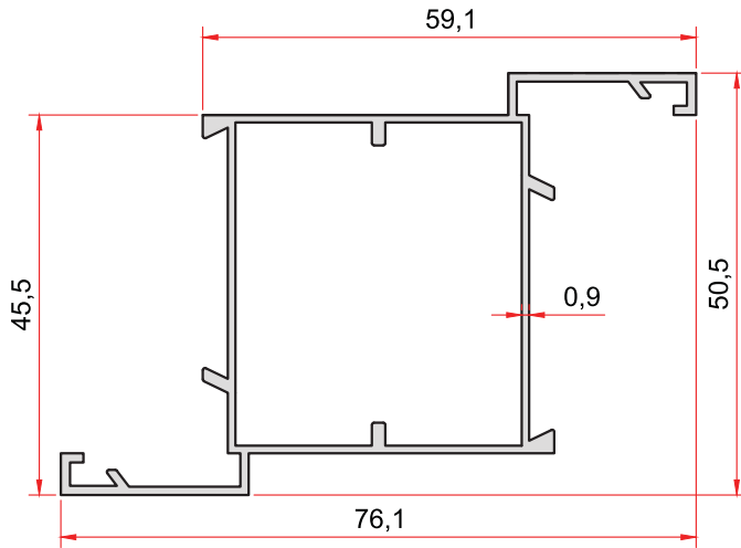
KOD-CODE TEORİK AĞIRLIK THEORETICAL WEIGHT EP-860 0,645 Kg/m
