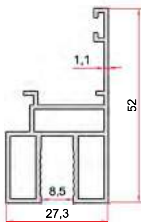
KOD-CODE TEORİK AĞIRLIK THEORETICAL WEIGHT EP-7043 0,583 Kg/m
