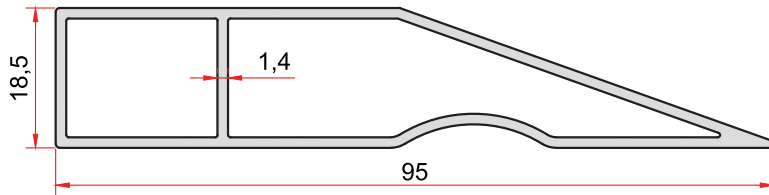
KOD-CODE TEORİK AĞIRLIK EP-4000 THEORETICAL WEIGHT 0,837 Kg/m
