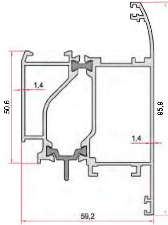
KOD-CODE TEORİK AĞIRLIK THEORETICAL WEIGHT EPİD-601-15 1,763 Kg/m
