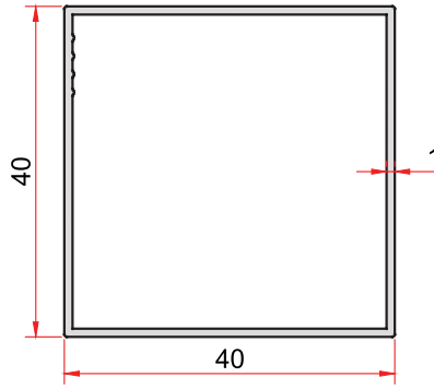
KOD-CODE TEORİK AĞIRLIK EP-773 THEORETICAL WEIGHT 0,421 Kg/m
