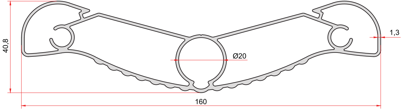
KOD-CODE TEORİK AĞIRLIK EP-4013 THEORETICAL WEIGHT 1,852 Kg/m
