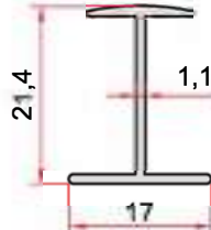
KOD-CODE TEORİK AĞIRLIK THEORETICAL WEIGHT EP-1385 0,140 Kg/m
