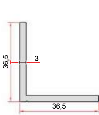
KOD-CODE TEORİK AĞIRLIK THEORETICAL WEIGHT EP-0776 0,567 Kg/m
