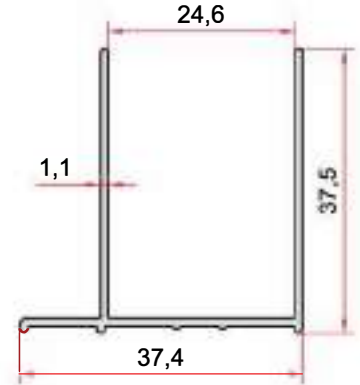
KOD-CODE TEORİK AĞIRLIK EP-1774 0,321 Kg/m
