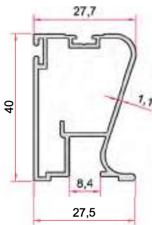
KOD-CODE TEORİK AĞIRLIK THEORETICAL WEIGHT EP-1393 0,505 Kg/m
