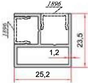
KOD-CODE TEORİK AĞIRLIK THEORETICAL WEIGHT EP-5063 0,335 Kg/m
