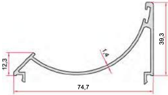
KOD-CODE TEORİK AĞIRLIK THEORETICAL WEIGHT EP-1202 0,621 Kg/m
