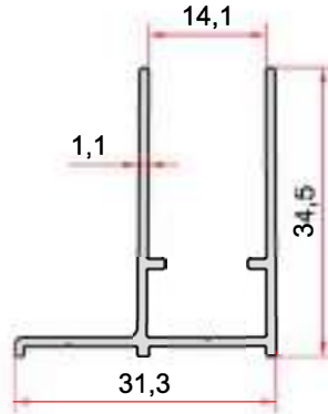
KOD-CODE TEORİK AĞIRLIK EP-1768 0,308 Kg/m
