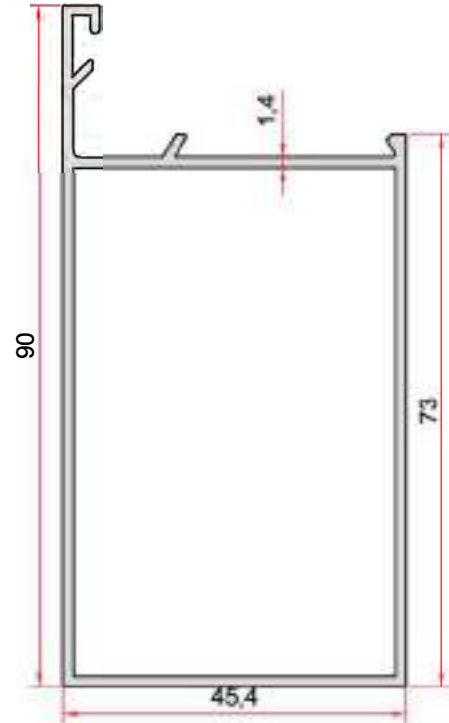
KOD-CODE TEORİK AĞIRLIK EP-0829 0,985 Kg/m
