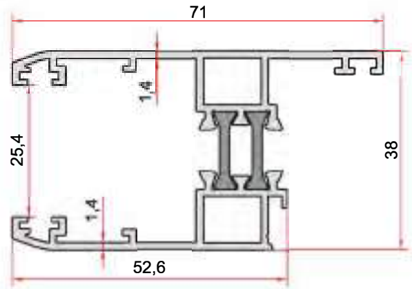
KOD-CODE TEORİK AĞIRLIK THEORETICAL WEIGHT EPİS-201-14 1,068 Kg/m
