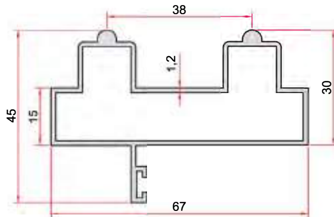
KOD-CODE TEORİK AĞIRLIK THEORETICAL WEIGHT EP-0816 0,810 Kg/m
