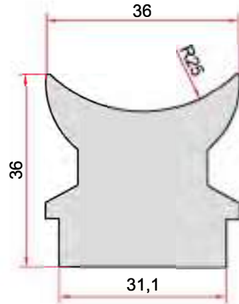
KOD-CODE TEORİK AĞIRLIK EP-1970 2,549 Kg/m
