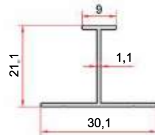
KOD-CODE TEORİK AĞIRLIK THEORETICAL WEIGHT EP-1378 0,173 Kg/m
