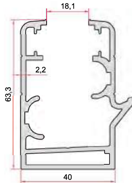
KOD-CODE TEORİK AĞIRLIK THEORETICAL WEIGHT EP-2272 1,545 Kg/m
