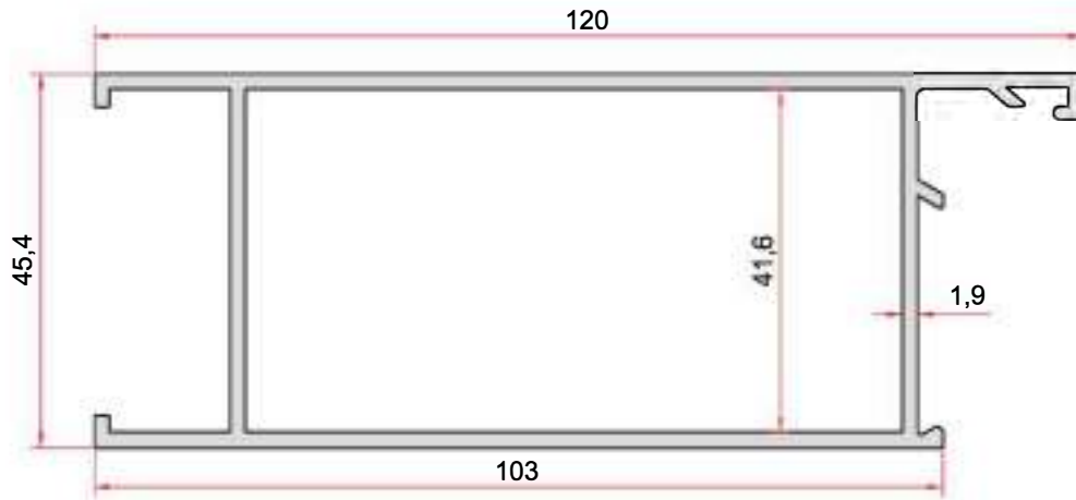
KOD-CODE TEORİK AĞIRLIK EP-0883 THEORETICAL WEIGHT 1,642 Kg/m
