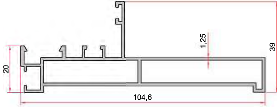
KOD-CODE TEORİK AĞIRLIK EP-1076 THEORETICAL WEIGHT 1,032 Kg/m
