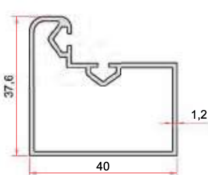
KOD-CODE TEORİK AĞIRLIK THEORETICAL WEIGHT EP-2294 0,540 Kg/m
