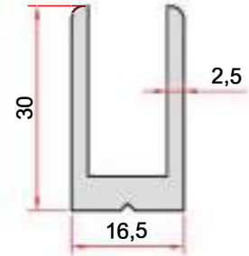
KOD-CODE TEORİK AĞIRLIK THEORETICAL WEIGHT EP-0841 0,553 Kg/m
