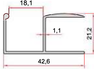
KOD-CODE TEORİK AĞIRLIK THEORETICAL WEIGHT EP-1403 0,346 Kg/m
