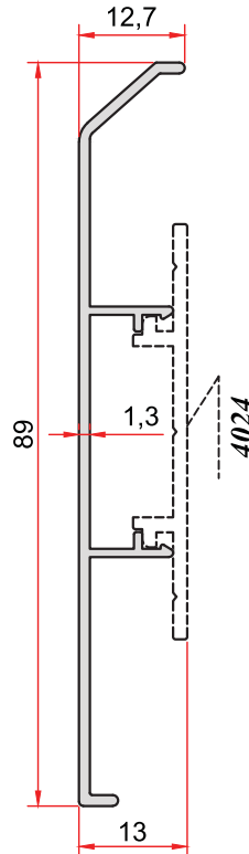
KOD-CODE TEORİK AĞIRLIK EP-4026 THEORETICAL WEIGHT 0,410 Kg/m
