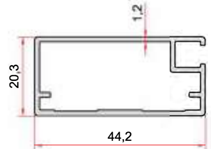
KOD-CODE TEORİK AĞIRLIK THEORETICAL WEIGHT EP-1462 0,467 Kg/m
