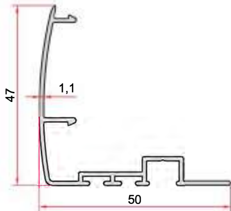
KOD-CODE TEORİK AĞIRLIK THEORETICAL WEIGHT EPSS-602-11 0,402 Kg/m
