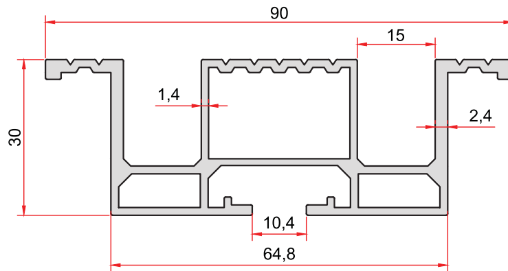
KOD-CODE TEORİK AĞIRLIK THEORETICAL WEIGHT EP- 6502 1,368 Kg/m
