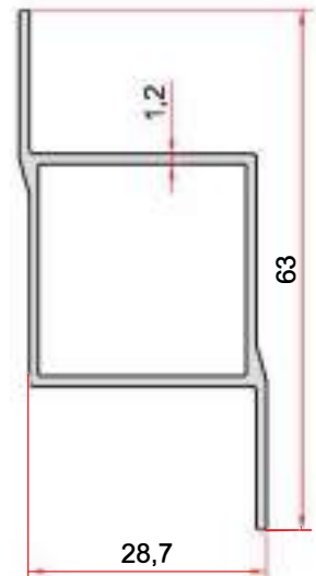
KOD-CODE TEORİK AĞIRLIK THEORETICAL WEIGHT EP-1018 0,475 Kg/m
