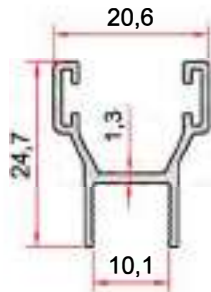
KOD-CODE TEORİK AĞIRLIK THEORETICAL WEIGHT EP-2376 0,224 Kg/m
