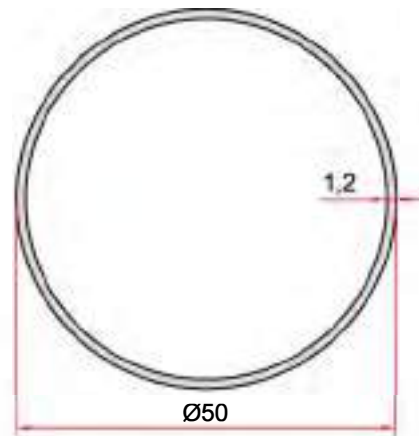
KOD-CODE TEORİK AĞIRLIK EP-5059 THEORETICAL WEIGHT 0,496 Kg/m
