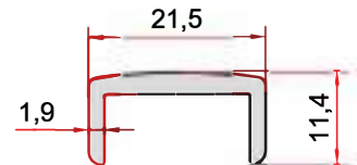
KOD-CODE TEORİK AĞIRLIK THEORETICAL WEIGHT EP-1122 0,229 Kg/m
