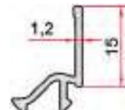
KOD-CODE TEORİK AĞIRLIK THEORETICAL WEIGHT EP-1206 0,119 Kg/m
