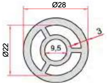
KOD-CODE TEORİK AĞIRLIK EP-5070 0,899 Kg/m THEORETICAL WEIGHT
