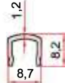
KOD-CODE TEORİK AĞIRLIK THEORETICAL WEIGHT EP-5101 0,062 Kg/m
