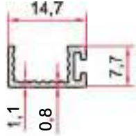
KOD-CODE TEORİK AĞIRLIK THEORETICAL WEIGHT EP-2720 0,092 Kg/m
