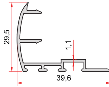
KOD-CODE TEORİK AĞIRLIK EP-787 THEORETICAL WEIGHT 0,305 Kg/m
