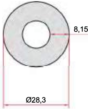
KOD-CODE TEORİK AĞIRLIK THEORETICAL WEIGHT EP-5029 1,393 Kg/m
