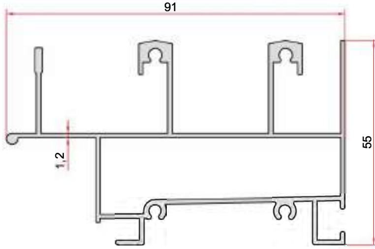
KOD-CODE TEORİK AĞIRLIK EP-7004 THEORETICAL WEIGHT 1,358 Kg/m
