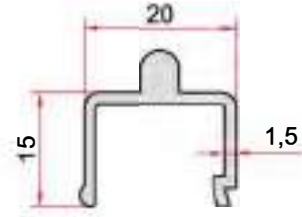
KOD-CODE TEORİK AĞIRLIK THEORETICAL WEIGHT EP-0810 0,262 Kg/m
