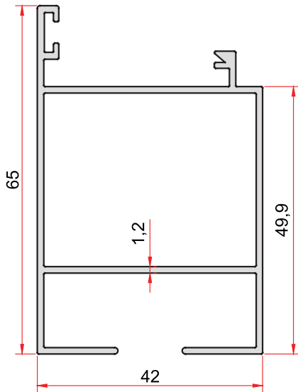
KOD-CODE TEORİK AĞIRLIK THEORETICAL WEIGHT EP-782 0,788 Kg/m
