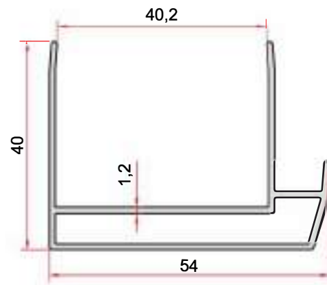
KOD-CODE TEORİK AĞIRLIK THEORETICAL WEIGHT EP-2619 0,610 Kg/m
