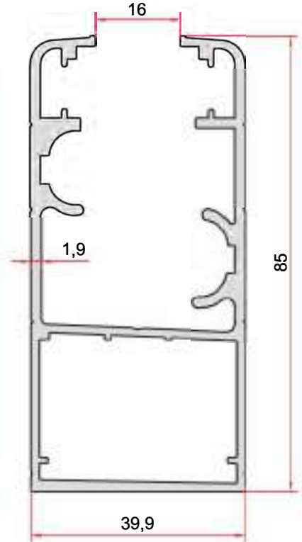
KOD-CODE TEORİK AĞIRLIK THEORETICAL WEIGHT EP-2730 1,547 Kg/m
