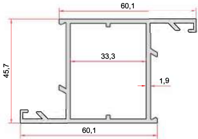
KOD-CODE TEORİK AĞIRLIK EP-0881 THEORETICAL WEIGHT 1,177 Kg/m
