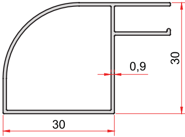
KOD-CODE TEORİK AĞIRLIK EP-772 THEORETICAL WEIGHT 0,337 Kg/m
