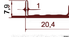
KOD-CODE TEORİK AĞIRLIK THEORETICAL WEIGHT EP-1506 0,090 Kg/m
