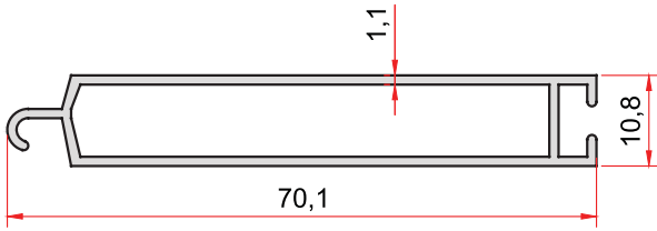
KOD-CODE TEORİK AĞIRLIK EP-2303 THEORETICAL WEIGHT 0,470 Kg/m
