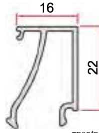
KOD-CODE TEORİK AĞIRLIK THEORETICAL WEIGHT EPCC-1160-13 0,260 Kg/m
