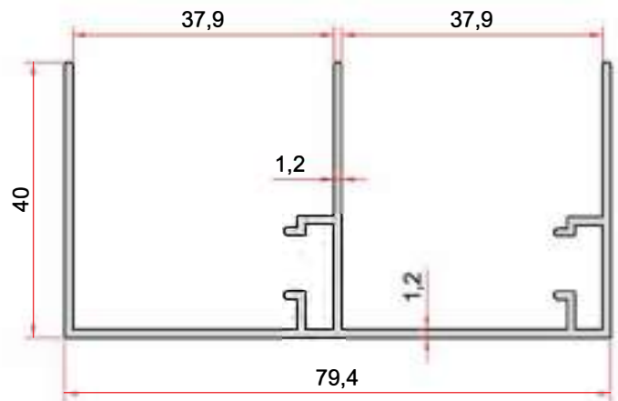
KOD-CODE TEORİK AĞIRLIK THEORETICAL WEIGHT EP-1489 0,737 Kg/m
