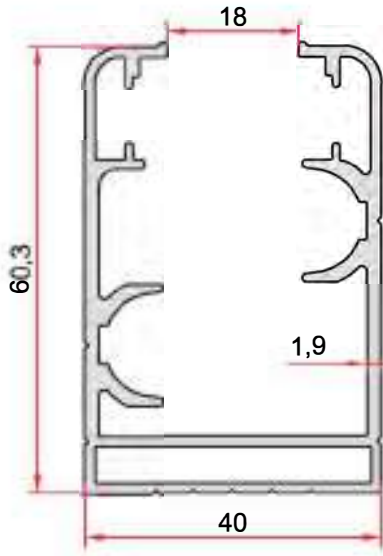
KOD-CODE EP-2762 TEORİK AĞIRLIK THEORETICAL WEIGHT 1,163 Kg/m
