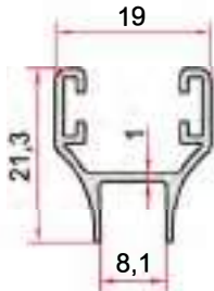
KOD-CODE TEORİK AĞIRLIK THEORETICAL WEIGHT EP-1429 0,197 Kg/m
