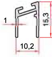
KOD-CODE TEORİK AĞIRLIK THEORETICAL WEIGHT EP-2391 0,116 Kg/m
