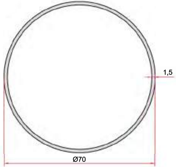
KOD-CODE TEORİK AĞIRLIK EP-5050 THEORETICAL WEIGHT 0,872 Kg/m
