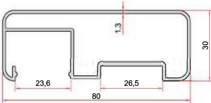
KOD-CODE TEORİK AĞIRLIK THEORETICAL WEIGHT EP-5006 0,915 Kg/m
