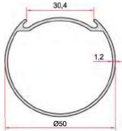
KOD-CODE TEORİK AĞIRLIK EP-5030 THEORETICAL WEIGHT 0,543 Kg/m
