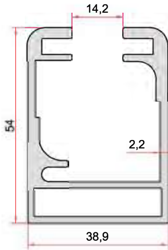
KOD-CODE EP-2270 TEORİK AĞIRLIK THEORETICAL WEIGHT 1,404 Kg/m
