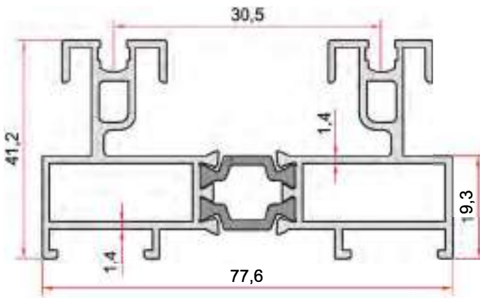
KOD-CODE TEORİK AĞIRLIK THEORETICAL WEIGHT EPİS-101-14 1,572 Kg/m
