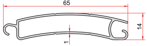
KOD-CODE TEORİK AĞIRLIK EP-2316 THEORETICAL WEIGHT 0,410 Kg/m
