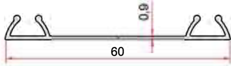
KOD-CODE TEORİK AĞIRLIK EP-1450 THEORETICAL WEIGHT 0,224 Kg/m
