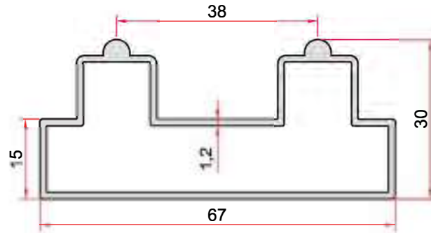
KOD-CODE TEORİK AĞIRLIK THEORETICAL WEIGHT EP-0898 0,732 Kg/m
