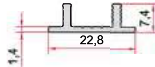
KOD-CODE TEORİK AĞIRLIK THEORETICAL WEIGHT EP-1025 0,153 Kg/m
