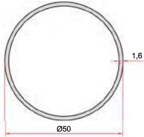
KOD-CODE TEORİK AĞIRLIK THEORETICAL WEIGHT EP-1912 0,656 Kg/m
