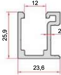
KOD-CODE TEORİK AĞIRLIK THEORETICAL WEIGHT EP-1959 0,475 Kg/m
