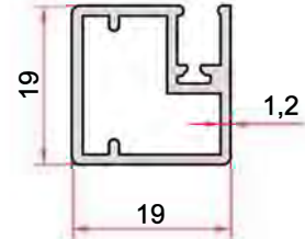
KOD-CODE TEORİK AĞIRLIK THEORETICAL WEIGHT EP-1426 0,294 Kg/m
