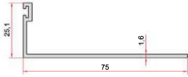
KOD-CODE TEORİK AĞIRLIK THEORETICAL WEIGHT EP-0155 0,454 Kg/m
