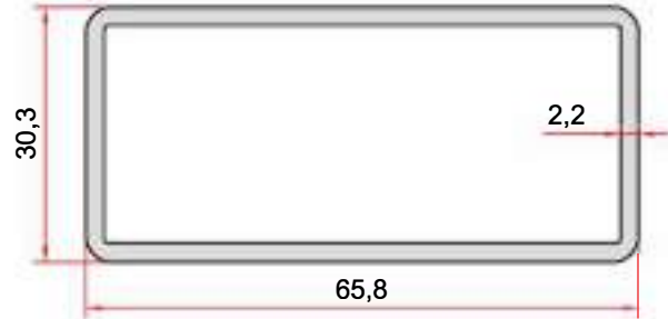
KOD-CODE TEORİK AĞIRLIK THEORETICAL WEIGHT EP-1972 1,069 Kg/m
