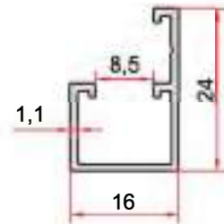
KOD-CODE TEORİK AĞIRLIK THEORETICAL WEIGHT EP-5080 0,180 Kg/m
