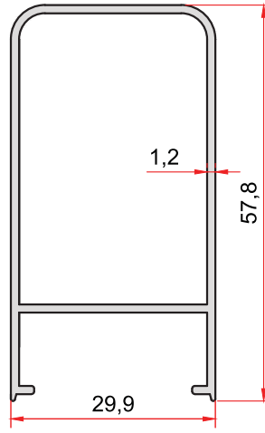
KOD-CODE TEORİK AĞIRLIK THEORETICAL WEIGHT EP-875 0,551 Kg/m
