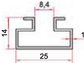
KOD-CODE TEORİK AĞIRLIK THEORETICAL WEIGHT EP-1391 0,197 Kg/m
