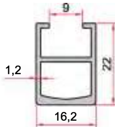
KOD-CODE TEORİK AĞIRLIK THEORETICAL WEIGHT EP-1950 0,273 Kg/m
