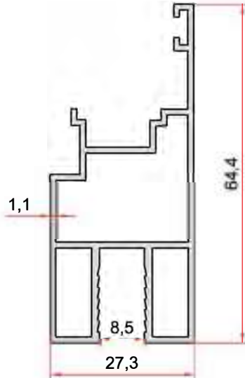
KOD-CODE TEORİK AĞIRLIK THEORETICAL WEIGHT EP-7042 0,696 Kg/m
