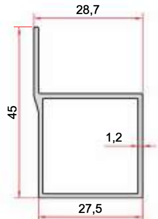
KOD-CODE TEORİK AĞIRLIK THEORETICAL WEIGHT EP-1017 0,406 Kg/m
