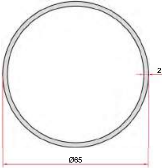
KOD-CODE TEORİK AĞIRLIK EP-1913 THEORETICAL WEIGHT 1,069 Kg/m
