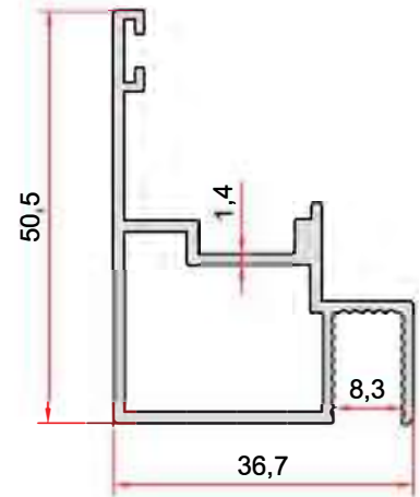
KOD-CODE TEORİK AĞIRLIK THEORETICAL WEIGHT EP-2681 0,610 Kg/m
