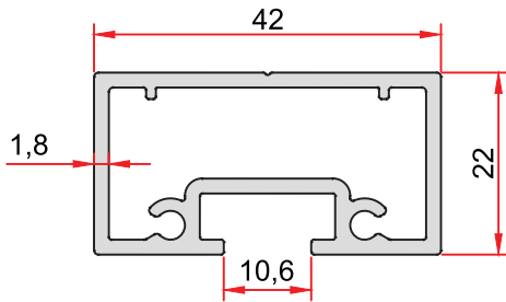
KOD-CODE TEORİK AĞIRLIK EPAO-1027-18 THEORETICAL WEIGHT 0,736 Kg/m
