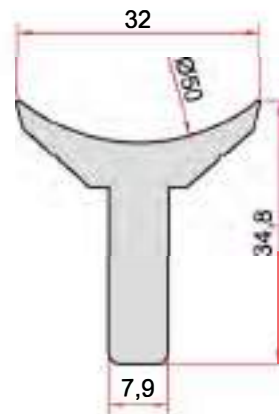
KOD-CODE TEORİK AĞIRLIK EP-1892 0,934 Kg/m
