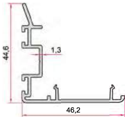
KOD-CODE TEORİK AĞIRLIK THEORETICAL WEIGHT EPSS-404-13 0,468 Kg/m
