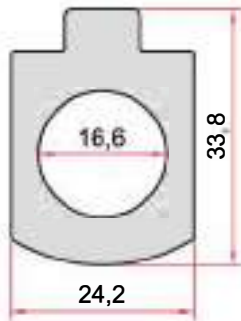
KOD-CODE TEORİK AĞIRLIK THEORETICAL WEIGHT EP-1855 1,337 Kg/m
