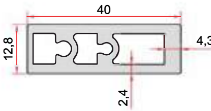
KOD-CODE TEORİK AĞIRLIK THEORETICAL WEIGHT EP-1499 0,797 Kg/m
