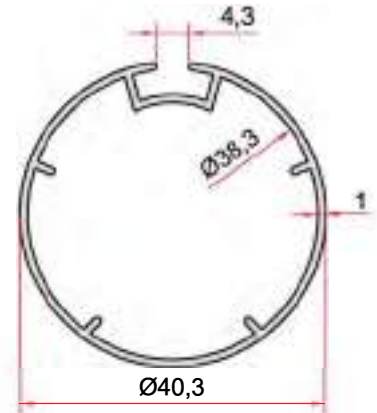
KOD-CODE TEORİK AĞIRLIK THEORETICAL WEIGHT EP-2213 0,397 Kg/m
