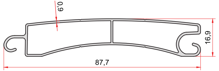
KOD-CODE TEORİK AĞIRLIK EP-2301 THEORETICAL WEIGHT 0,572 Kg/m
