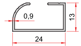
KOD-CODE TEORİK AĞIRLIK EP-779 THEORETICAL WEIGHT 0,143 Kg/m
