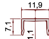
KOD-CODE TEORİK AĞIRLIK THEORETICAL WEIGHT EP-1896 0,065 Kg/m
