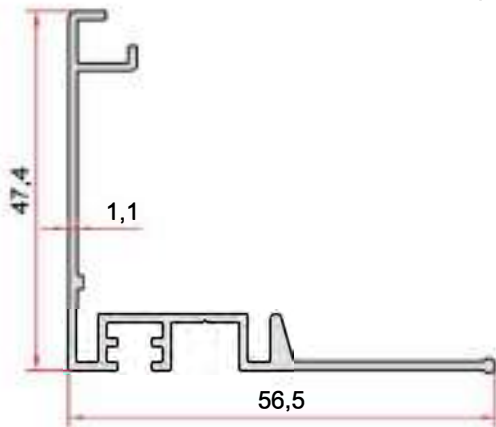
KOD-CODE TEORİK AĞIRLIK EPMD-102-11 THEORETICAL WEIGHT 0,461 Kg/m
