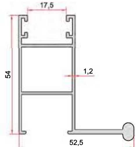
KOD-CODE TEORİK AĞIRLIK EP-1014 THEORETICAL WEIGHT 0,776 Kg/m
