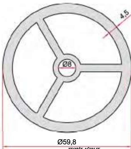
KOD-CODE TEORİK AĞIRLIK EP-1870 2,870 Kg/m THEORETICAL WEIGHT
