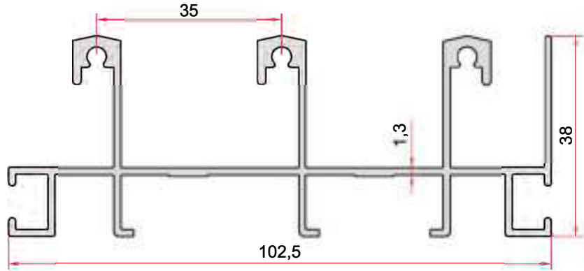
KOD-CODE TEORİK AĞIRLIK EP-1007 THEORETICAL WEIGHT 1,320 Kg/m
