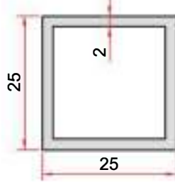
KOD-CODE TEORİK AĞIRLIK THEORETICAL WEIGHT EP-0053 0,497 Kg/m
