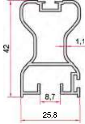
KOD-CODE TEORİK AĞIRLIK THEORETICAL WEIGHT EP-1365 0,516 Kg/m
