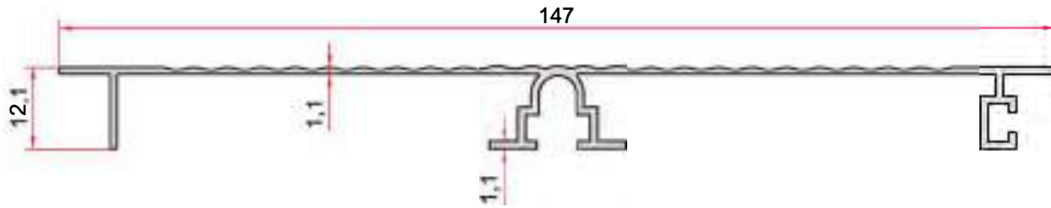
KOD-CODE TEORİK AĞIRLIK THEORETICAL WEIGHT EP-1353 0,588 Kg/m
