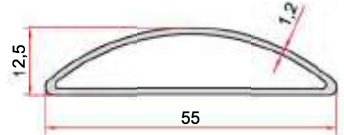
KOD-CODE TEORİK AĞIRLIK THEORETICAL WEIGHT EP-5058 0,371 Kg/m
