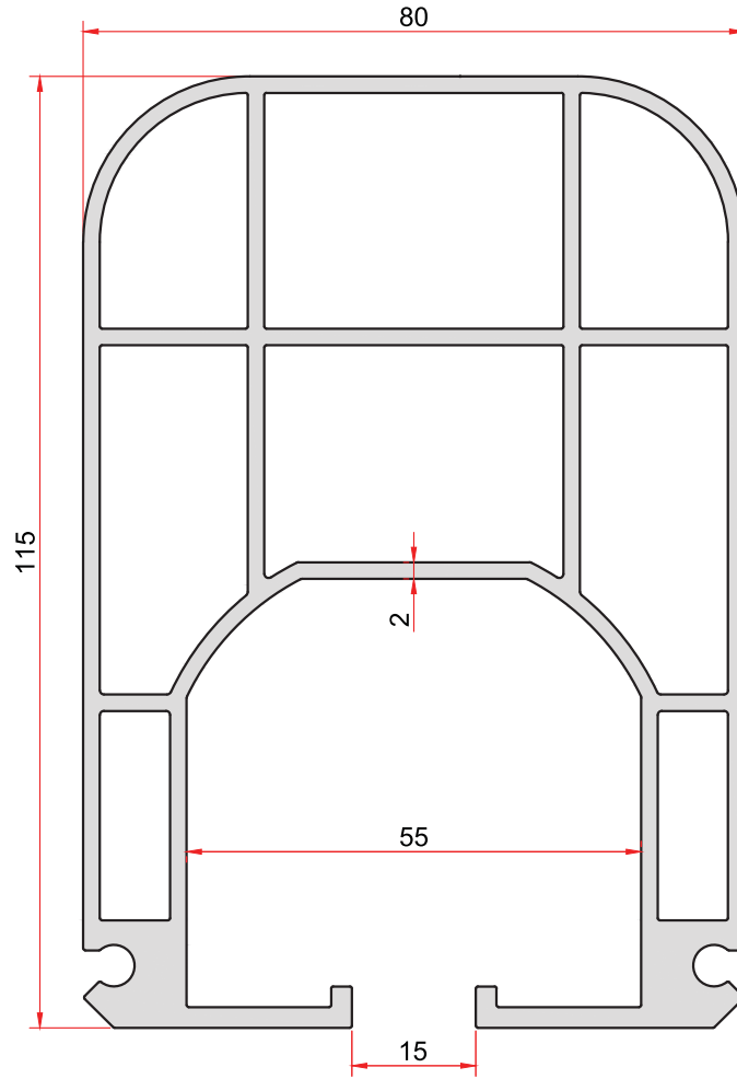
KOD-CODE TEORİK AĞIRLIK EP-0097 THEORETICAL WEIGHT 4,222 Kg/m
