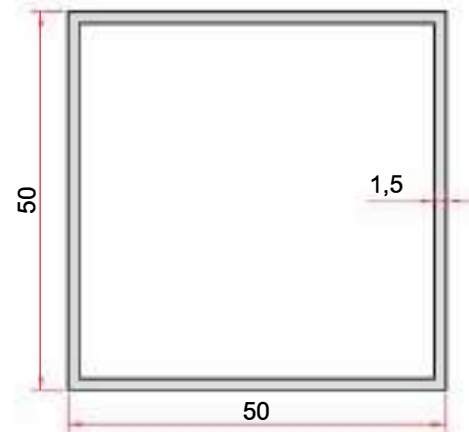
KOD-CODE TEORİK AĞIRLIK THEORETICAL WEIGHT EP-0119 0,785 Kg/m
