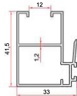
KOD-CODE TEORİK AĞIRLIK EP-1005 THEORETICAL WEIGHT 0,575 Kg/m
