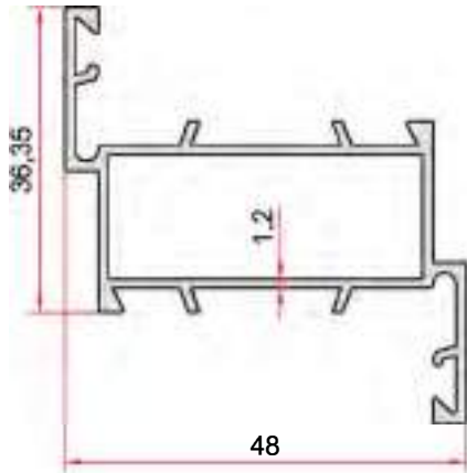
KOD-CODE TEORİK AĞIRLIK THEORETICAL WEIGHT EP-1012 0,632 Kg/m
