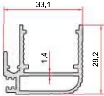
KOD-CODE TEORİK AĞIRLIK THEORETICAL WEIGHT EP-2677 0,526 Kg/m
