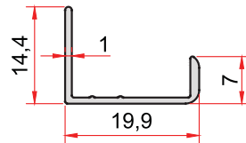
KOD-CODE TEORİK AĞIRLIK EP-778 THEORETICAL WEIGHT 0,103 Kg/m
