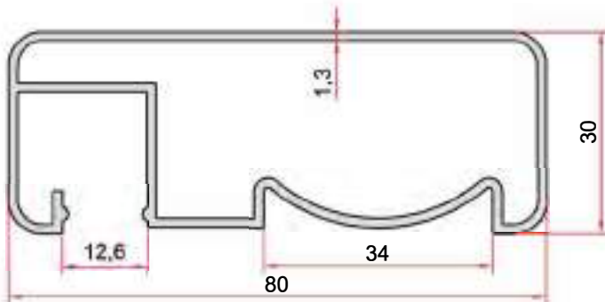
KOD-CODE TEORİK AĞIRLIK THEORETICAL WEIGHT EP-5007 0,915 Kg/m
