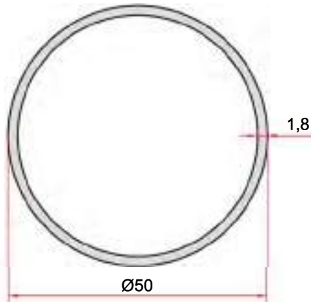
KOD-CODE TEORİK AĞIRLIK THEORETICAL WEIGHT EP-1921 0,737 Kg/m
