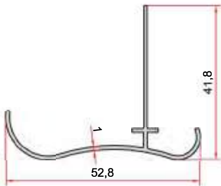
KOD-CODE TEORİK AĞIRLIK THEORETICAL WEIGHT EP-1242 0,297 Kg/m
