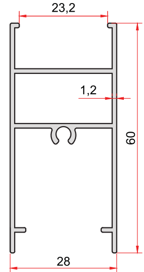
KOD-CODE TEORİK AĞIRLIK THEORETICAL WEIGHT EP- 876 0,610 Kg/m
