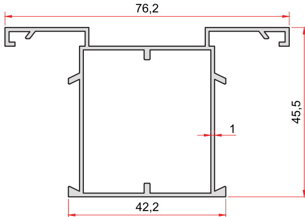
KOD-CODE TEORİK AĞIRLIK THEORETICAL WEIGHT EP-856 0,683 Kg/m
