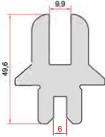
KOD-CODE TEORİK AĞIRLIK EP-1856 2,530 Kg/m
