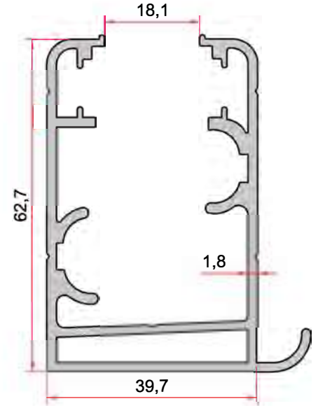
KOD-CODE TEORİK AĞIRLIK THEORETICAL WEIGHT EP-2450 1,378 Kg/m
