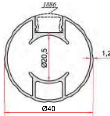
KOD-CODE TEORİK AĞIRLIK THEORETICAL WEIGHT EP-1904 0,580 Kg/m
