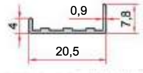
KOD-CODE TEORİK AĞIRLIK THEORETICAL WEIGHT EP-1392 0,081 Kg/m
