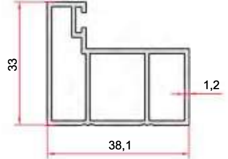
KOD-CODE TEORİK AĞIRLIK THEORETICAL WEIGHT EP-2731 0,578 Kg/m
