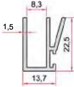
KOD-CODE TEORİK AĞIRLIK THEORETICAL WEIGHT EP-2443 0,300 Kg/m
