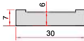
KOD-CODE TEORİK AĞIRLIK EP-1428 THEORETICAL WEIGHT 0,510 Kg/m
