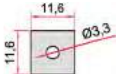
KOD-CODE TEORİK AĞIRLIK THEORETICAL WEIGHT EP-1499 0,797 Kg/m
