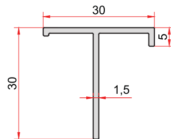
KOD-CODE TEORİK AĞIRLIK EP-1060 THEORETICAL WEIGHT 0,254 Kg/m
