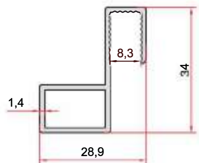
KOD-CODE TEORİK AĞIRLIK THEORETICAL WEIGHT EP-2682 0,375 Kg/m
