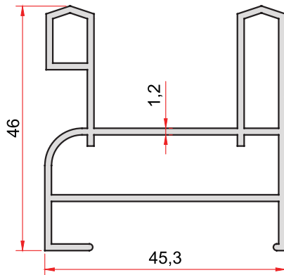
KOD-CODE TEORİK AĞIRLIK EP-788 THEORETICAL WEIGHT 0,802 Kg/m
