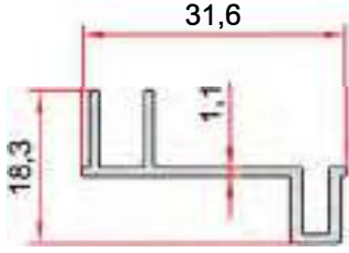
KOD-CODE TEORİK AĞIRLIK EP-1789 0,207 Kg/m
