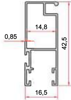
KOD-CODE TEORİK AĞIRLIK THEORETICAL WEIGHT EP-1310 0,335 Kg/m
