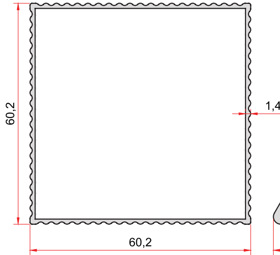
KOD-CODE TEORİK AĞIRLIK EP-4015 THEORETICAL WEIGHT 0,702 Kg/m
