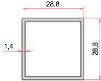
KOD-CODE TEORİK AĞIRLIK THEORETICAL WEIGHT EP-5083 0,413 Kg/m
