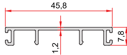
KOD-CODE TEORİK AĞIRLIK THEORETICAL WEIGHT EPAO-1043-12 0,261 Kg/m
