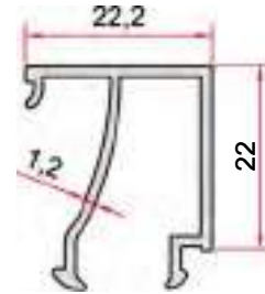
KOD-CODE TEORİK AĞIRLIK THEORETICAL WEIGHT EPİS-302-15 0,286 Kg/m
