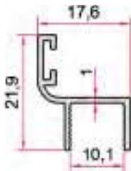
KOD-CODE TEORİK AĞIRLIK THEORETICAL WEIGHT EP-2377 0,151 Kg/m
