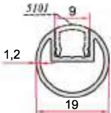
KOD-CODE TEORİK AĞIRLIK THEORETICAL WEIGHT EP-5100 0,218 Kg/m
