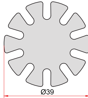
KOD-CODE TEORİK AĞIRLIK THEORETICAL WEIGHT EP-5094 2,438 Kg/m
