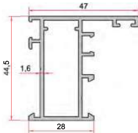
KOD-CODE TEORİK AĞIRLIK EP-1089 0,826 Kg/m
