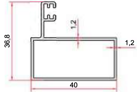
KOD-CODE TEORİK AĞIRLIK THEORETICAL WEIGHT EP-2726 0,472 Kg/m
