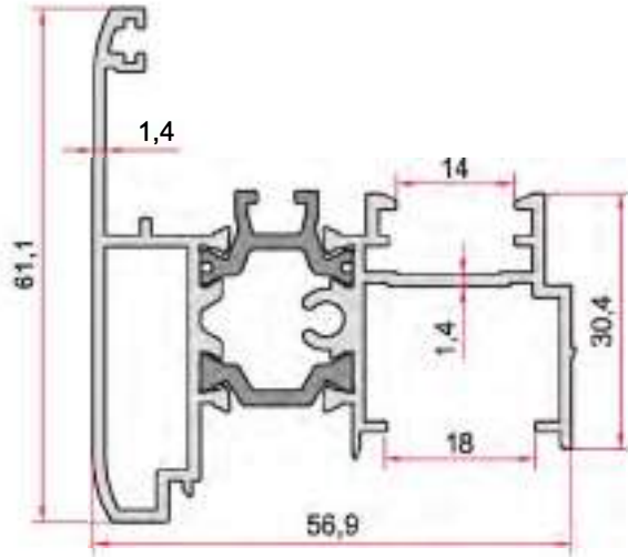
KOD-CODE TEORİK AĞIRLIK THEORETICAL WEIGHT EPİD-701-14 1,213 Kg/m
