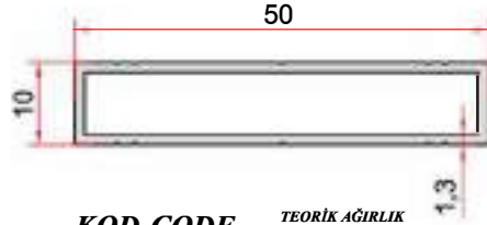
KOD-CODE TEORİK AĞIRLIK THEORETICAL WEIGHT EP-5088 0,400 Kg/m
