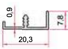
KOD-CODE TEORİK AĞIRLIK THEORETICAL WEIGHT EP-1356 0,097 Kg/m
