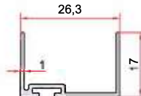
KOD-CODE TEORİK AĞIRLIK THEORETICAL WEIGHT EP-2758 0,180 Kg/m
