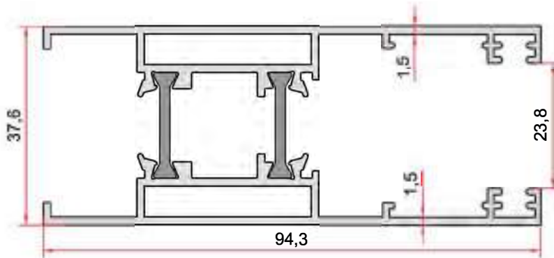
KOD-CODE TEORİK AĞIRLIK EPMD-101-15 THEORETICAL WEIGHT 1,616 Kg/m
