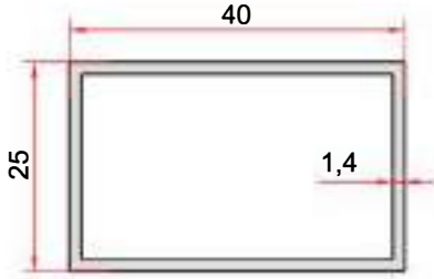
KOD-CODE TEORİK AĞIRLIK THEORETICAL WEIGHT EP-5078 0,470 Kg/m
