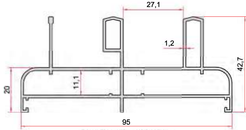
KOD-CODE TEORİK AĞIRLIK THEORETICAL WEIGHT EP-1134 1,218 Kg/m
