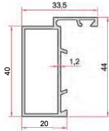
KOD-CODE TEORİK AĞIRLIK EP-1074 0,494 Kg/m
