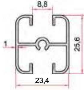
KOD-CODE TEORİK AĞIRLIK THEORETICAL WEIGHT EP-1362 0,316 Kg/m
