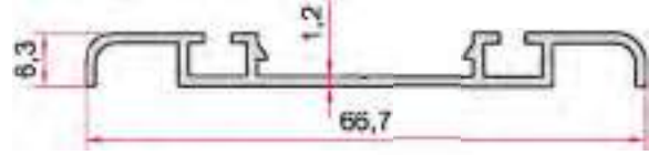
KOD-CODE TEORİK AĞIRLIK EP-1355 THEORETICAL WEIGHT 0,337 Kg/m
