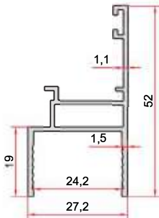
KOD-CODE TEORİK AĞIRLIK THEORETICAL WEIGHT EP-2755 0,434 Kg/m
