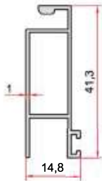
KOD-CODE TEORİK AĞIRLIK THEORETICAL WEIGHT EP-7010 0,313 Kg/m
