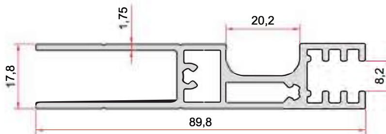
KOD-CODE TEORİK AĞIRLIK THEORETICAL WEIGHT EP-2444 1,226 Kg/m
