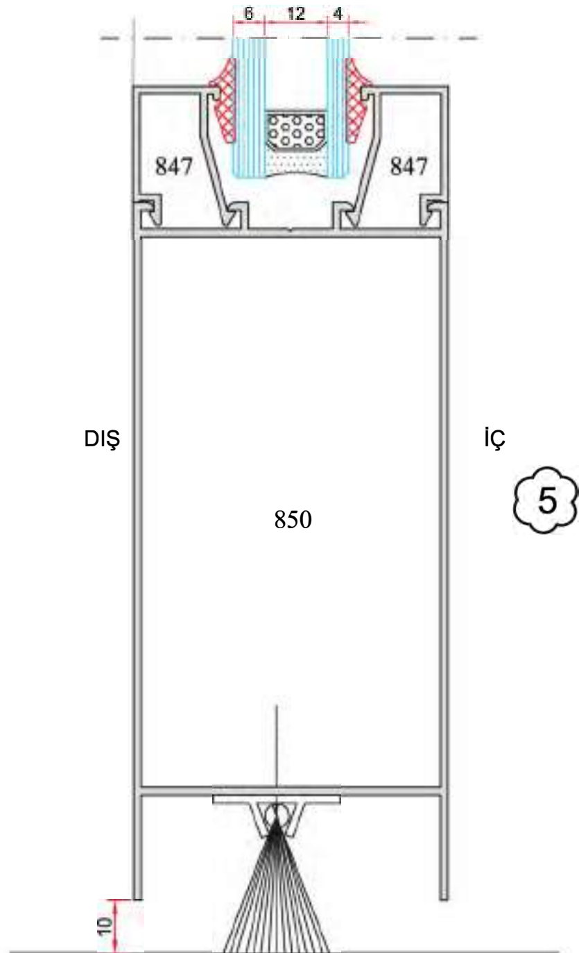
İÇE AÇILIR KAPI DOOR - INSIDE OPENING
