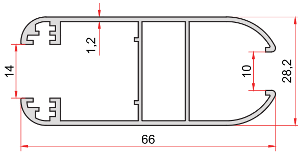
KOD-CODE TEORİK AĞIRLIK EP-785 THEORETICAL WEIGHT 0,726 Kg/m
