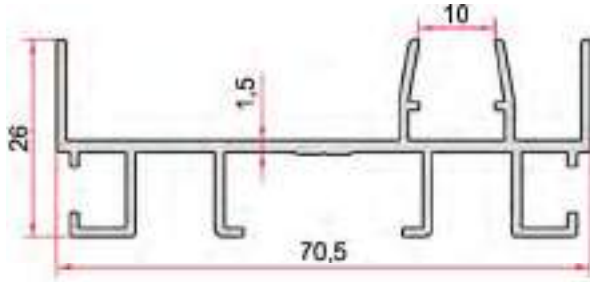
KOD-CODE TEORİK AĞIRLIK THEORETICAL WEIGHT EP-1022 0,705 Kg/m
