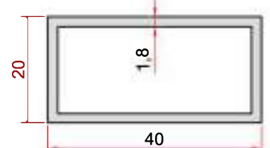
KOD-CODE TEORİK AĞIRLIK THEORETICAL WEIGHT EP-0031 0,548 Kg/m
