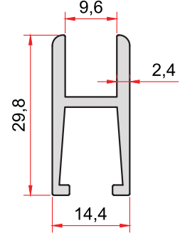
KOD-CODE TEORİK AĞIRLIK THEORETICAL WEIGHT EP-0501 0,396 Kg/m
