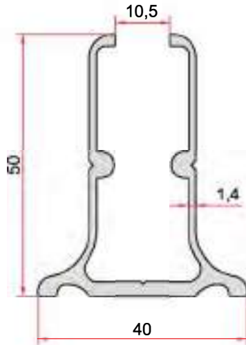
KOD-CODE TEORİK AĞIRLIK THEORETICAL WEIGHT EP-5039 0,756 Kg/m
