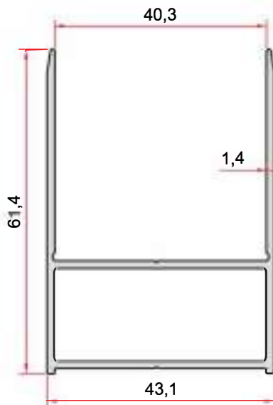
KOD-CODE EP-2267 TEORİK AĞIRLIK THEORETICAL WEIGHT 0,759 Kg/m
