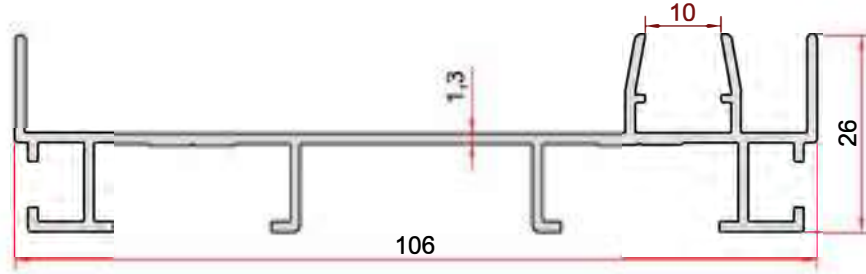
KOD-CODE TEORİK AĞIRLIK EP-1024 THEORETICAL WEIGHT 0,859 Kg/m
