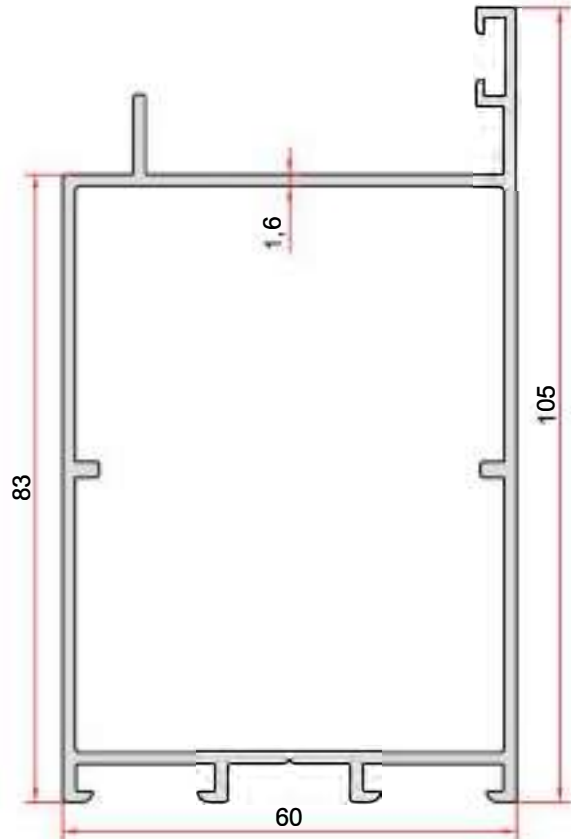
KOD-CODE TEORİK AĞIRLIK EP-1241 1,493 Kg/m
