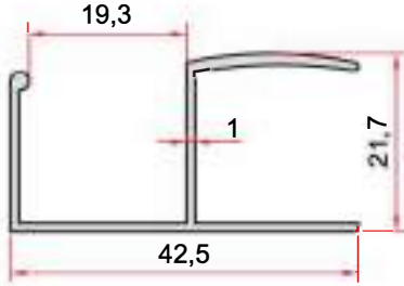
KOD-CODE TEORİK AĞIRLIK THEORETICAL WEIGHT EP-1387 0,294 Kg/m
