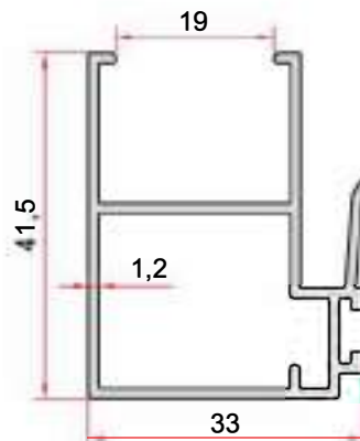
KOD-CODE TEORİK AĞIRLIK EP-1003 THEORETICAL WEIGHT 0,540 Kg/m
