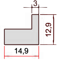
KOD-CODE TEORİK AĞIRLIK THEORETICAL WEIGHT EP-1409 0,319 Kg/m
