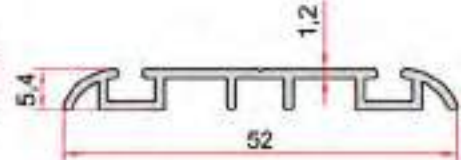
KOD-CODE TEORİK AĞIRLIK THEORETICAL WEIGHT EP-1372 0,275 Kg/m
