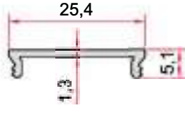
KOD-CODE TEORİK AĞIRLIK THEORETICAL WEIGHT EP-1354 0,121 Kg/m
