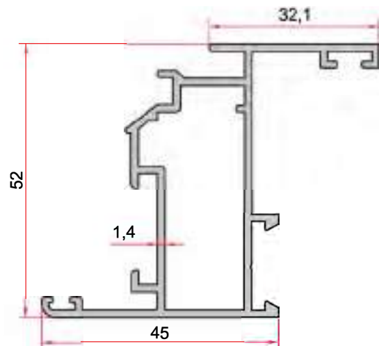
KOD-CODE TEORİK AĞIRLIK EP-1085 0,875 Kg/m
