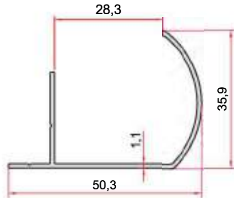
KOD-CODE TEORİK AĞIRLIK EP-1756 0,313 Kg/m
