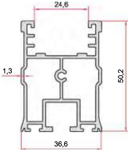
KOD-CODE TEORİK AĞIRLIK EP-2751 THEORETICAL WEIGHT 0,980 Kg/m
