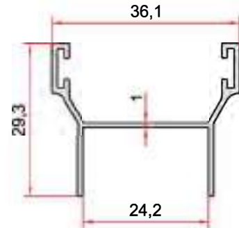
KOD-CODE TEORİK AĞIRLIK THEORETICAL WEIGHT EP-2759 0,272 Kg/m
