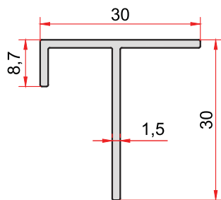
KOD-CODE TEORİK AĞIRLIK EP-1059 THEORETICAL WEIGHT 0,265 Kg/m
