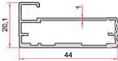
KOD-CODE TEORİK AĞIRLIK THEORETICAL WEIGHT EP-1460 0,410 Kg/m
