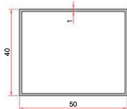
KOD-CODE TEORİK AĞIRLIK THEORETICAL WEIGHT EP-0035 0,475 Kg/m
