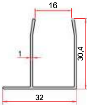
KOD-CODE TEORİK AĞIRLIK EP-1767 0,243 Kg/m
