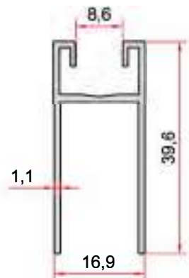
KOD-CODE TEORİK AĞIRLIK THEORETICAL WEIGHT EP-1400 0,324 Kg/m
