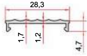
KOD-CODE TEORİK AĞIRLIK THEORETICAL WEIGHT EP-2696 0,125 Kg/m
