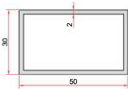
KOD-CODE TEORİK AĞIRLIK THEORETICAL WEIGHT EP-0054 0,821 Kg/m
