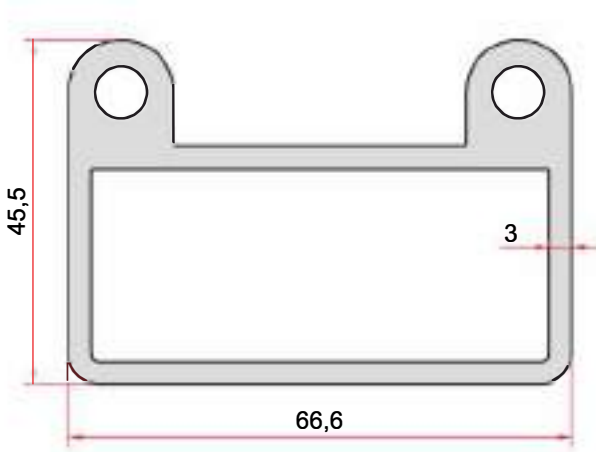
KOD-CODE TEORİK AĞIRLIK THEORETICAL WEIGHT EP-1983 2,217 Kg/m
