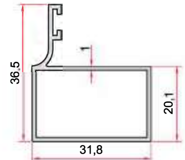
KOD-CODE TEORİK AĞIRLIK THEORETICAL WEIGHT EP-2262 0,359 Kg/m
