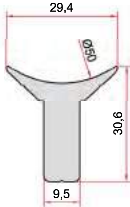
KOD-CODE TEORİK AĞIRLIK EP-1942 0,853 Kg/m
