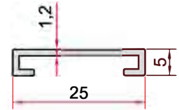
KOD-CODE TEORİK AĞIRLIK THEORETICAL WEIGHT EP-0837 0,124 Kg/m
