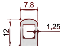
KOD-CODE TEORİK AĞIRLIK THEORETICAL WEIGHT EP-1494 0,156 Kg/m
