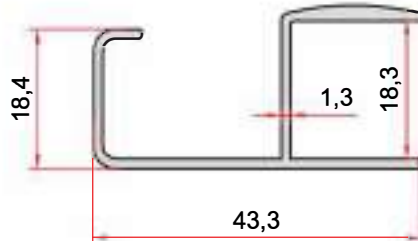
KOD-CODE TEORİK AĞIRLIK THEORETICAL WEIGHT EP-1507 0,367 Kg/m
