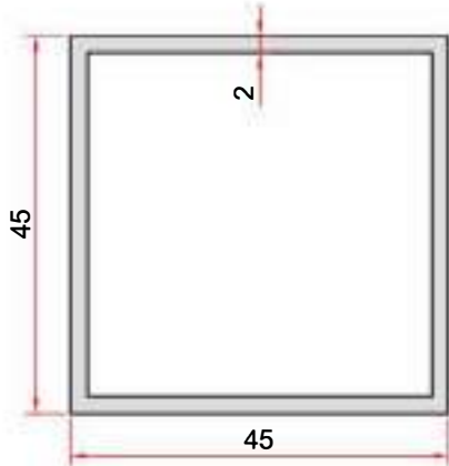
KOD-CODE TEORİK AĞIRLIK THEORETICAL WEIGHT EP-0061 0,929 Kg/m
