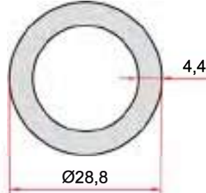
KOD-CODE TEORİK AĞIRLIK THEORETICAL WEIGHT EP-1894 0,910 Kg/m
