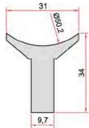
KOD-CODE TEORİK AĞIRLIK EP-1862 1,007 Kg/m
