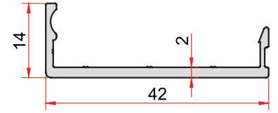
KOD-CODE TEORİK AĞIRLIK EP-4012 THEORETICAL WEIGHT 0,292 Kg/m
