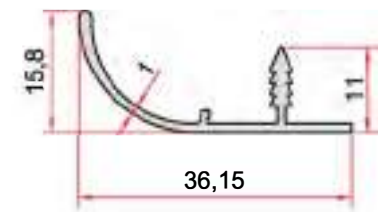
KOD-CODE TEORİK AĞIRLIK THEORETICAL WEIGHT EP-1484 0,211 Kg/m
