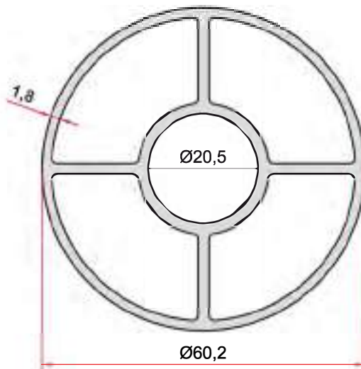
KOD-CODE TEORİK AĞIRLIK EP-1858 1,628 Kg/m THEORETICAL WEIGHT
