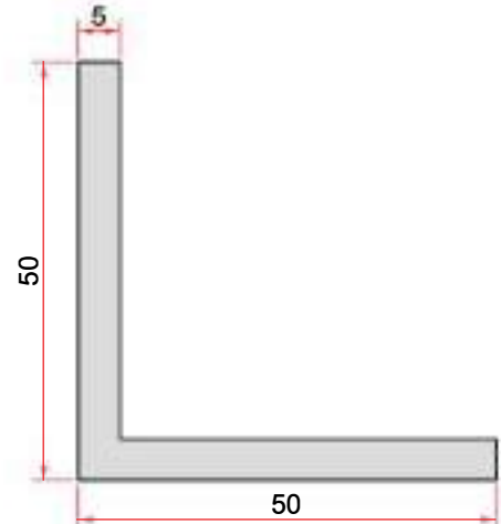
KOD-CODE TEORİK AĞIRLIK THEORETICAL WEIGHT EP-0022 1,282 Kg/m
