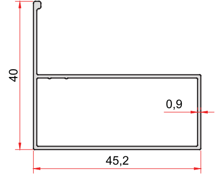
KOD-CODE TEORİK AĞIRLIK EP-771 THEORETICAL WEIGHT 0,364 Kg/m
