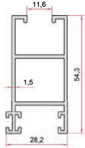
KOD-CODE TEORİK AĞIRLIK EP-1071 THEORETICAL WEIGHT 0,762 Kg/m
