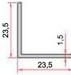
KOD-CODE TEORİK AĞIRLIK EP-0135 THEORETICAL WEIGHT 0,184 Kg/m
