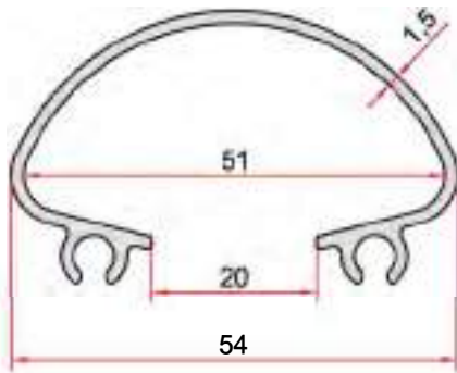
KOD-CODE TEORİK AĞIRLIK THEORETICAL WEIGHT EP-5051 0,548 Kg/m
