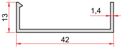
KOD-CODE TEORİK AĞIRLIK EP-4003 THEORETICAL WEIGHT 0,248 Kg/m
