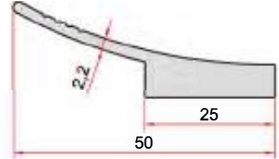
KOD-CODE TEORİK AĞIRLIK THEORETICAL WEIGHT EP-1471 0,645 Kg/m
