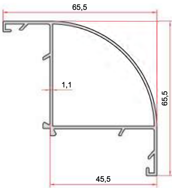
KOD-CODE TEORİK AĞIRLIK EP-0838 THEORETICAL WEIGHT 0,699 Kg/m
