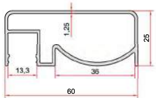
KOD-CODE TEORİK AĞIRLIK THEORETICAL WEIGHT EP-1961 0,675 Kg/m
