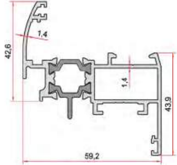
KOD-CODE TEORİK AĞIRLIK THEORETICAL WEIGHT EPİD-401-14 1,197 Kg/m
