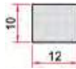
KOD-CODE TEORİK AĞIRLIK EP-1413 THEORETICAL WEIGHT 0,324 Kg/m
