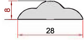
KOD-CODE TEORİK AĞIRLIK THEORETICAL WEIGHT EP-1444 0,389 Kg/m
