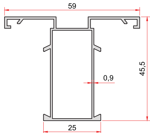
KOD-CODE TEORİK AĞIRLIK THEORETICAL WEIGHT EP-862 0,537 Kg/m
