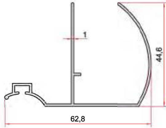
KOD-CODE TEORİK AĞIRLIK THEORETICAL WEIGHT EP-1784 0,451 Kg/m
