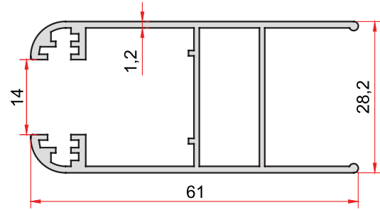
KOD-CODE TEORİK AĞIRLIK EP-786 THEORETICAL WEIGHT 0,667 Kg/m
