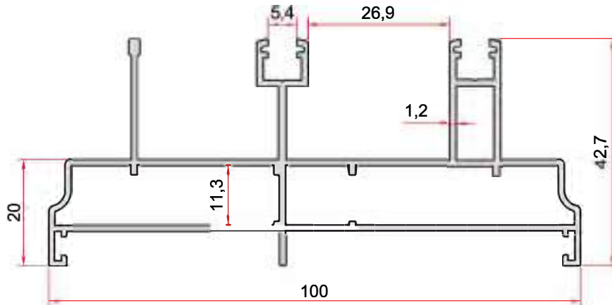
KOD-CODE TEORİK AĞIRLIK THEORETICAL WEIGHT EP-1139 1,188 Kg/m
