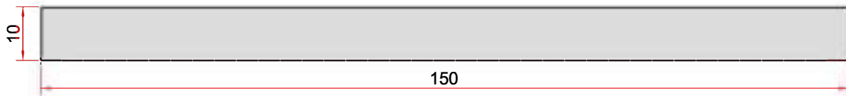
KOD-CODE TEORİK AĞIRLIK THEORETICAL WEIGHT EP-0134 4,050 Kg/m
