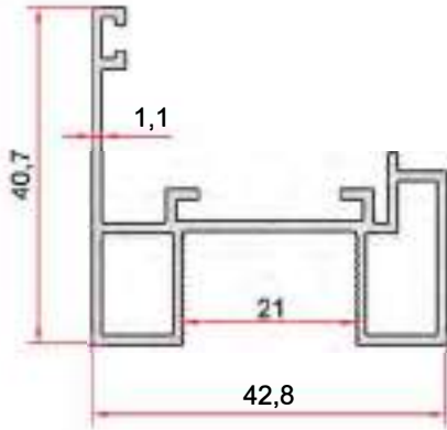
KOD-CODE TEORİK AĞIRLIK THEORETICAL WEIGHT EP-2732 0,529 Kg/m
