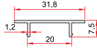
KOD-CODE TEORİK AĞIRLIK THEORETICAL WEIGHT EPAO-1041-12 0,145 Kg/m
