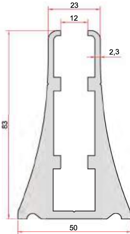
KOD-CODE TEORİK AĞIRLIK THEORETICAL WEIGHT EP-1879 3,226 Kg/m
