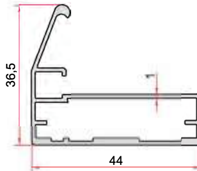
KOD-CODE TEORİK AĞIRLIK THEORETICAL WEIGHT EP-1461 0,475 Kg/m
