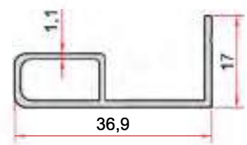
KOD-CODE TEORİK AĞIRLIK THEORETICAL WEIGHT EP-1430 0,267 Kg/m
