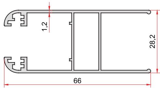
KOD-CODE TEORİK AĞIRLIK EP-851 THEORETICAL WEIGHT 0,699 Kg/m
