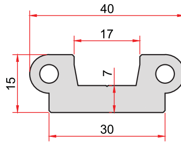
KOD-CODE TEORİK AĞIRLIK THEORETICAL WEIGHT EP-6501 0,975 Kg/m
