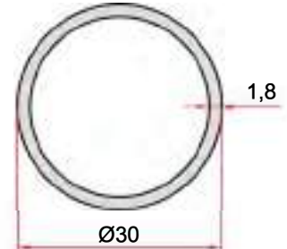
KOD-CODE TEORİK AĞIRLIK THEORETICAL WEIGHT EP-1911 0,429 Kg/m
