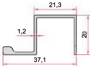
KOD-CODE TEORİK AĞIRLIK THEORETICAL WEIGHT EP-1374 0,281 Kg/m
