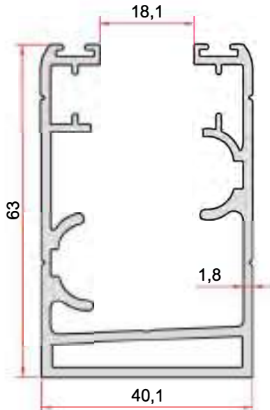
KOD-CODE TEORİK AĞIRLIK THEORETICAL WEIGHT EP-2371 1,328 Kg/m
