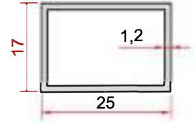
KOD-CODE TEORİK AĞIRLIK THEORETICAL WEIGHT EP-0114 0,256 Kg/m
