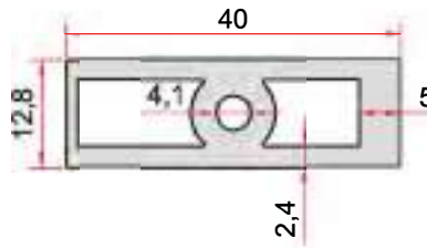
KOD-CODE TEORİK AĞIRLIK THEORETICAL WEIGHT EP-1493 0,807 Kg/m
