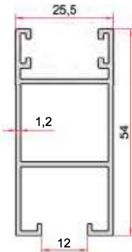
KOD-CODE TEORİK AĞIRLIK THEORETICAL WEIGHT EP-1002 0,605 Kg/m
