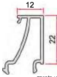
KOD-CODE TEORİK AĞIRLIK THEORETICAL WEIGHT EPCC-1120-13 0,254 Kg/m
