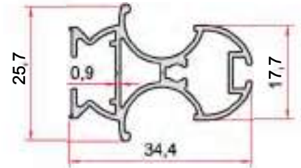
KOD-CODE TEORİK AĞIRLIK THEORETICAL WEIGHT EP-1755 0,385 Kg/m
