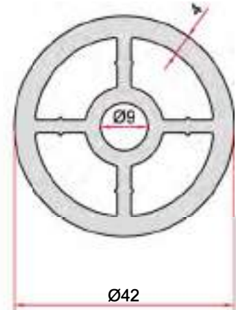
KOD-CODE TEORİK AĞIRLIK EP-1920 1,857 Kg/m THEORETICAL WEIGHT
