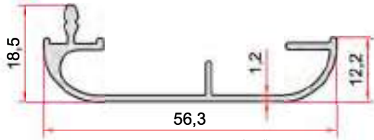
KOD-CODE TEORİK AĞIRLIK THEORETICAL WEIGHT EP-1038 0,373 Kg/m
