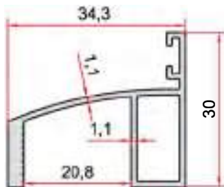
KOD-CODE TEORİK AĞIRLIK THEORETICAL WEIGHT EP-2750 0,383 Kg/m
