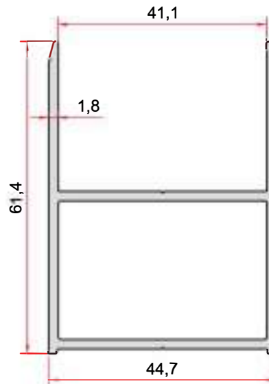
KOD-CODE EP-2253 TEORİK AĞIRLIK THEORETICAL WEIGHT 0,983 Kg/m
