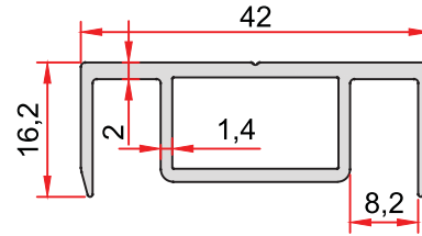
KOD-CODE TEORİK AĞIRLIK EPAO-1028-14 THEORETICAL WEIGHT 0,491 Kg/m
