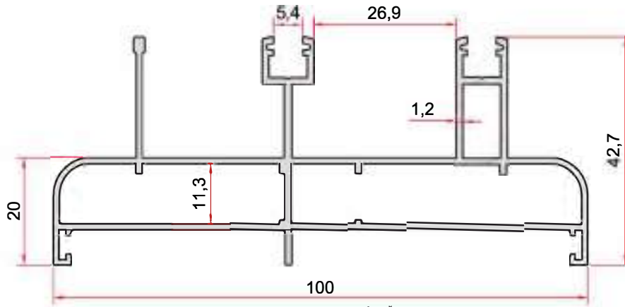
KOD-CODE TEORİK AĞIRLIK THEORETICAL WEIGHT EP-1138 1,182 Kg/m
