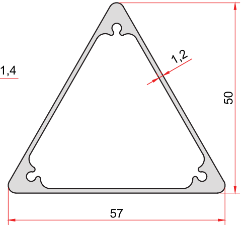
KOD-CODE TEORİK AĞIRLIK EP-4018 THEORETICAL WEIGHT 0,788 Kg/m
