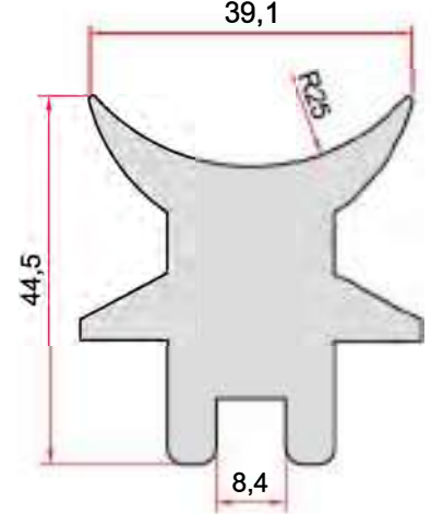
KOD-CODE TEORİK AĞIRLIK EP-1966 2,397 Kg/m
