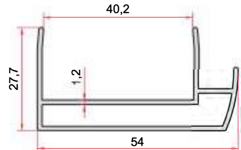
KOD-CODE TEORİK AĞIRLIK THEORETICAL WEIGHT EP-2392 0,532 Kg/m
