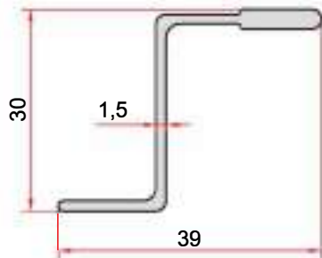
KOD-CODE TEORİK AĞIRLIK THEORETICAL WEIGHT EP-1308 0,413 Kg/m
