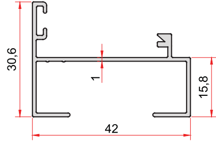
KOD-CODE TEORİK AĞIRLIK THEORETICAL WEIGHT EP-781 0,348 Kg/m
