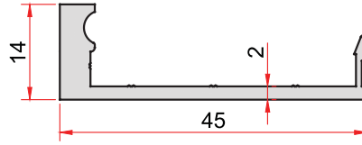
KOD-CODE TEORİK AĞIRLIK EP-4011 THEORETICAL WEIGHT 0,402 Kg/m
