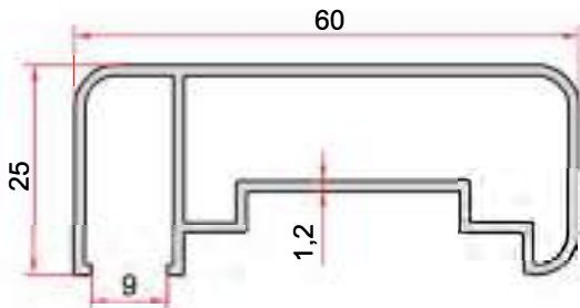
KOD-CODE TEORİK AĞIRLIK THEORETICAL WEIGHT EP-5079 0,607 Kg/m
