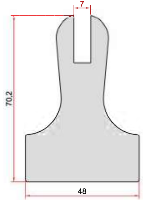
KOD-CODE TEORİK AĞIRLIK THEORETICAL WEIGHT EP-5046 5,054 Kg/m
