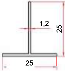
KOD-CODE TEORİK AĞIRLIK THEORETICAL WEIGHT EP-0019 0,157 Kg/m
