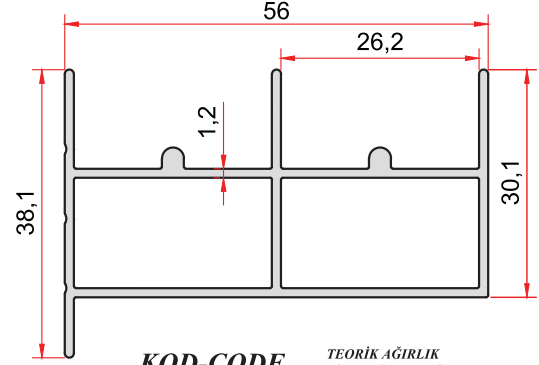
KOD-CODE TEORİK AĞIRLIK THEORETICAL WEIGHT EP-0100 0,693 Kg/m
