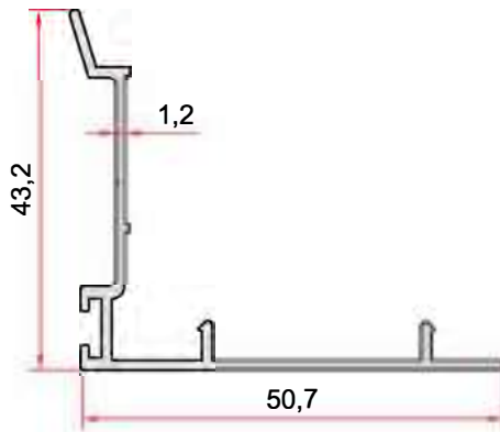
KOD-CODE TEORİK AĞIRLIK THEORETICAL WEIGHT EP-0809 0,370 Kg/m
