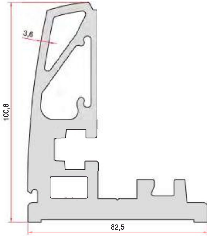
KOD-CODE TEORİK AĞIRLIK THEORETICAL WEIGHT EP-2277 5,918 Kg/m
