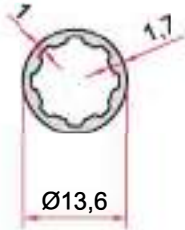
KOD-CODE TEORİK AĞIRLIK THEORETICAL WEIGHT EP-2217 0,140 Kg/m
