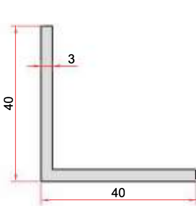
KOD-CODE TEORİK AĞIRLIK THEORETICAL WEIGHT EP-0145 0,623 Kg/m
