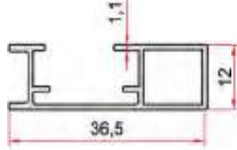
KOD-CODE TEORİK AĞIRLIK EP-1761 0,259 Kg/m
