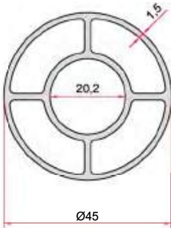
KOD-CODE TEORİK AĞIRLIK EP-5028 1,053 Kg/m THEORETICAL WEIGHT
