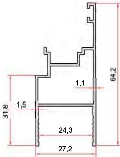
KOD-CODE TEORİK AĞIRLIK THEORETICAL WEIGHT EP-2754 0,545 Kg/m
