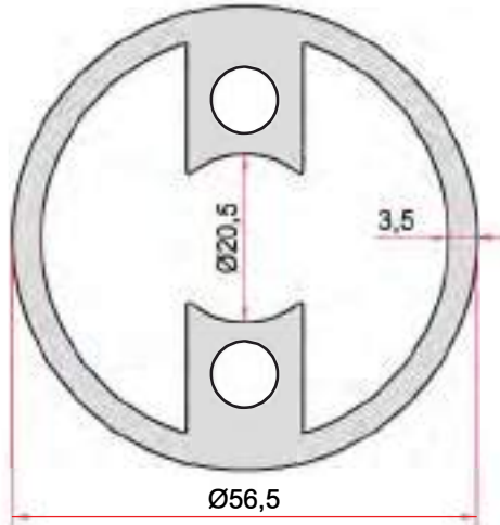
KOD-CODE TEORİK AĞIRLIK EP-1971 2,440 Kg/m THEORETICAL WEIGHT
