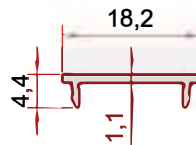
KOD-CODE TEORİK AĞIRLIK THEORETICAL WEIGHT EP-1142 0,068 Kg/m
