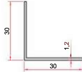
KOD-CODE TEORİK AĞIRLIK EP-0016 THEORETICAL WEIGHT 0,192 Kg/m
