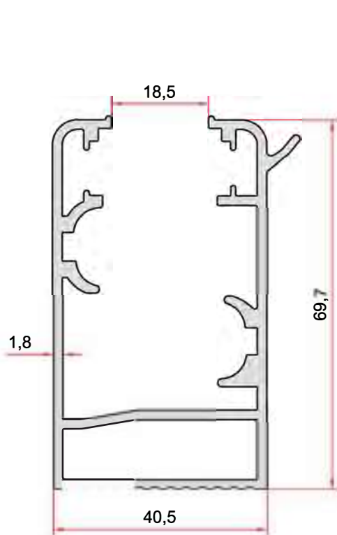
KOD-CODE TEORİK AĞIRLIK THEORETICAL WEIGHT EP-2752 1,441 Kg/m
