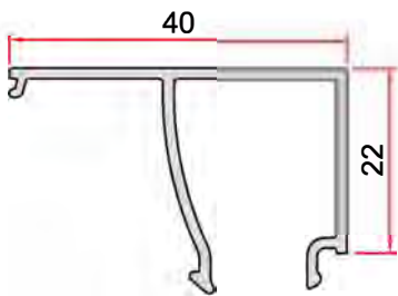
KOD-CODE TEORİK AĞIRLIK THEORETICAL WEIGHT EPCC-1400-13 0,341 Kg/m
