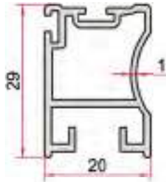
KOD-CODE TEORİK AĞIRLIK THEORETICAL WEIGHT EP-1397 0,394 Kg/m
