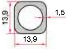
KOD-CODE TEORİK AĞIRLIK THEORETICAL WEIGHT EP-1906 0,248 Kg/m
