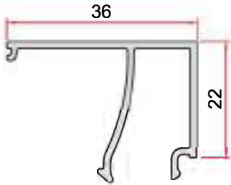
KOD-CODE TEORİK AĞIRLIK THEORETICAL WEIGHT EPCC-1360-13 0,327 Kg/m
