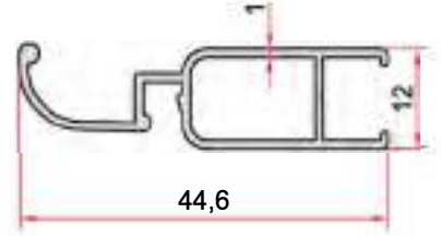
KOD-CODE TEORİK AĞIRLIK THEORETICAL WEIGHT EP-1303 0,286 Kg/m
