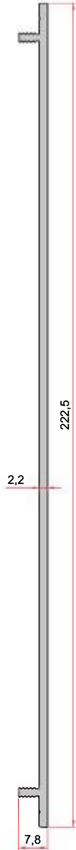
KOD-CODE TEORİK AĞIRLIK THEORETICAL WEIGHT EP-1094 1,388 Kg/m
