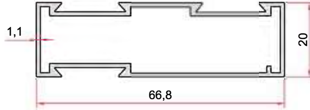
KOD-CODE TEORİK AĞIRLIK THEORETICAL WEIGHT EP-0885 0,599 Kg/m
