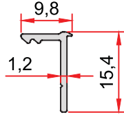
KOD-CODE TEORİK AĞIRLIK THEORETICAL WEIGHT EPAO-1032-13 0,078 Kg/m
