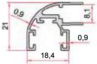
KOD-CODE TEORİK AĞIRLIK THEORETICAL WEIGHT EP-2265 0,265 Kg/m
