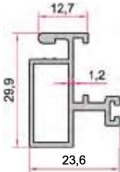
KOD-CODE TEORİK AĞIRLIK THEORETICAL WEIGHT EP-1072 0,397 Kg/m
