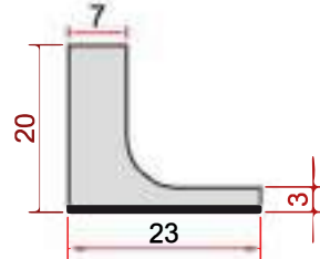
KOD-CODE TEORİK AĞIRLIK THEORETICAL WEIGHT EP-1414 0,529 Kg/m
