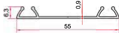
KOD-CODE TEORİK AĞIRLIK EP-1373 THEORETICAL WEIGHT 0,211 Kg/m
