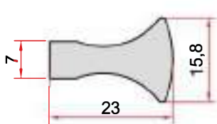
KOD-CODE TEORİK AĞIRLIK THEORETICAL WEIGHT EP-1439 0,489 Kg/m
