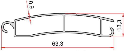
KOD-CODE TEORİK AĞIRLIK EP-2313 THEORETICAL WEIGHT 0,402 Kg/m
