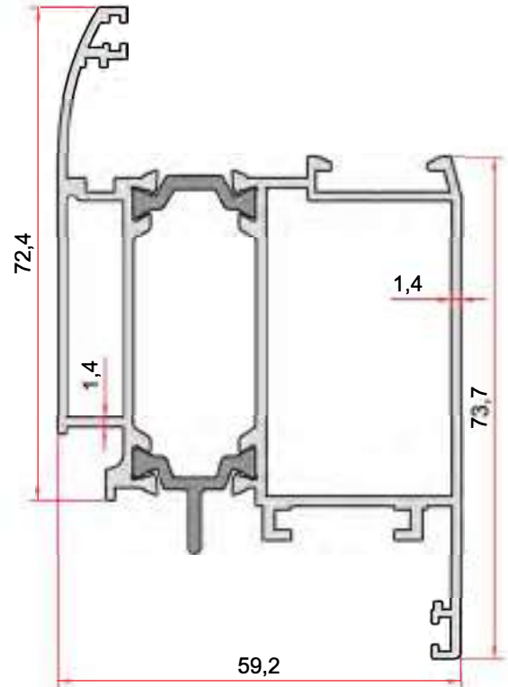
KOD-CODE TEORİK AĞIRLIK THEORETICAL WEIGHT EPİD-501-15 1,702 Kg/m
