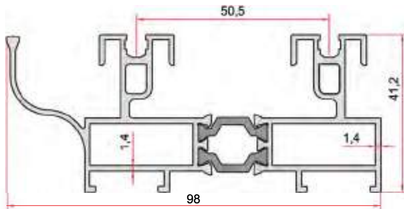
KOD-CODE TEORİK AĞIRLIK THEORETICAL WEIGHT EPİS-101-14 1,572 Kg/m
