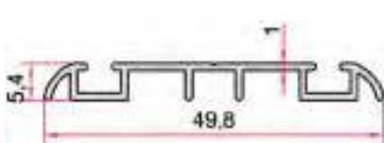
KOD-CODE TEORİK AĞIRLIK THEORETICAL WEIGHT EP-1456 0,230 Kg/m
