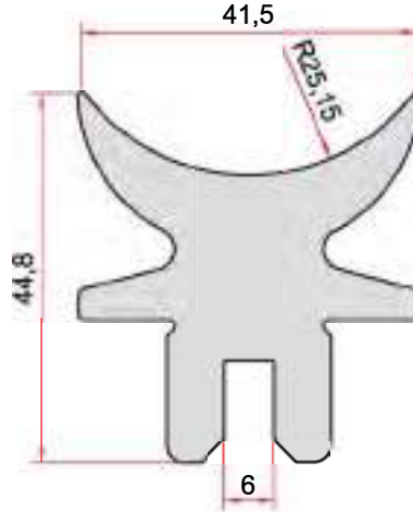
KOD-CODE TEORİK AĞIRLIK EP-1857 2,403 Kg/m
