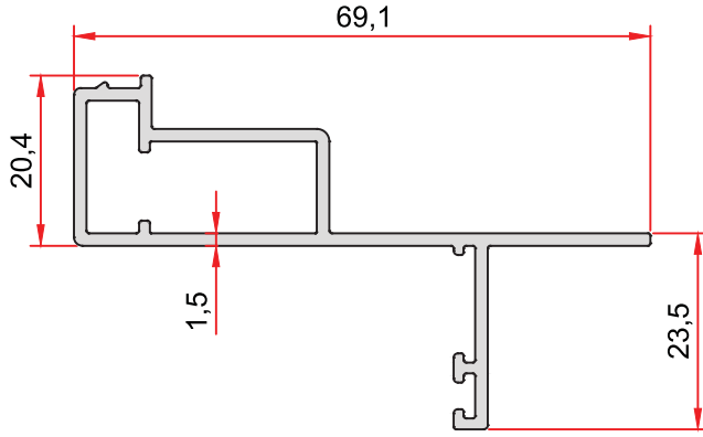
KOD-CODE TEORİK AĞIRLIK EPAO-1024-13 THEORETICAL WEIGHT 0,669 Kg/m
