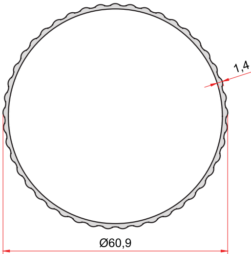
KOD-CODE TEORİK AĞIRLIK THEORETICAL WEIGHT EP- 4014 0,583 Kg/m
