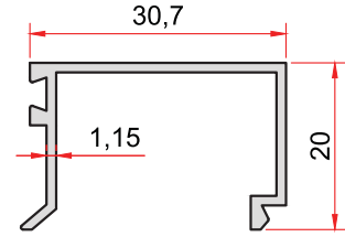
KOD-CODE TEORİK AĞIRLIK THEORETICAL WEIGHT EP-859 0,248 Kg/m
