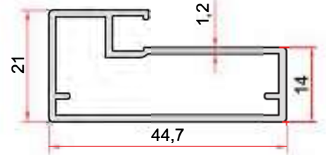
KOD-CODE TEORİK AĞIRLIK THEORETICAL WEIGHT EP-1381 0,475 Kg/m
