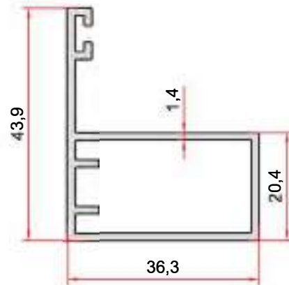
KOD-CODE TEORİK AĞIRLIK EP-2756 THEORETICAL WEIGHT 0,564 Kg/m
