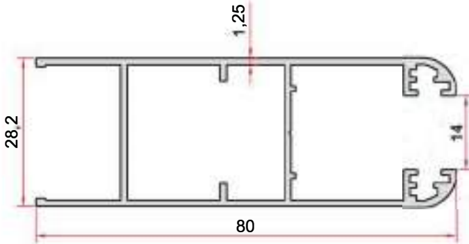
KOD-CODE TEORİK AĞIRLIK THEORETICAL WEIGHT EP-1135 0,848 Kg/m
