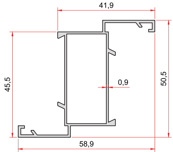
KOD-CODE TEORİK AĞIRLIK THEORETICAL WEIGHT EP-861 0,537 Kg/m
