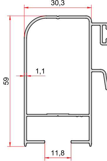
KOD-CODE TEORİK AĞIRLIK EP-770 THEORETICAL WEIGHT 0,643 Kg/m
