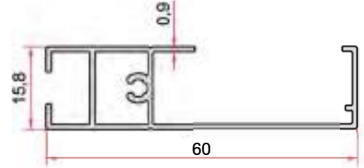
KOD-CODE TEORİK AĞIRLIK EP-1765 0,391 Kg/m
