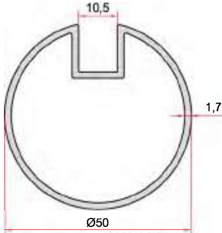
KOD-CODE TEORİK AĞIRLIK EP-1929 THEORETICAL WEIGHT 0,810 Kg/m
