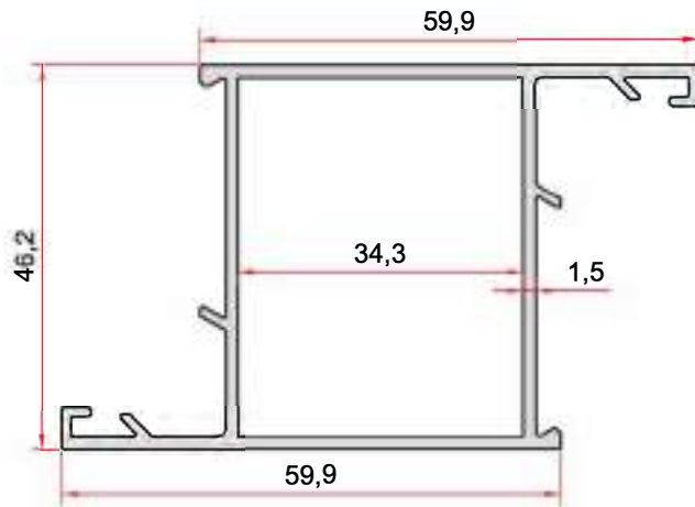
KOD-CODE TEORİK AĞIRLIK EP-0906 THEORETICAL WEIGHT 0,921 Kg/m
