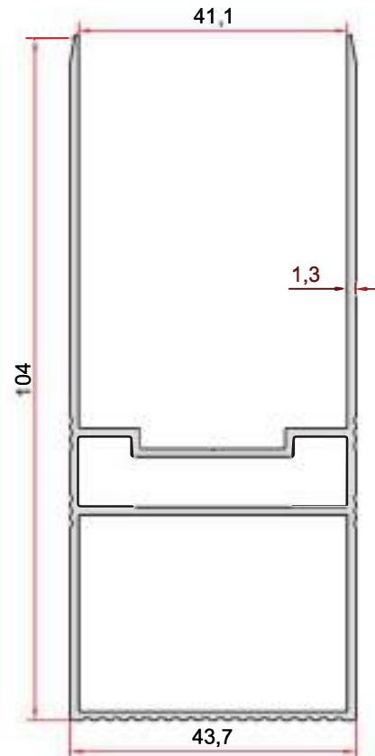
KOD-CODE TEORİK AĞIRLIK THEORETICAL WEIGHT EP-2663 1,150 Kg/m
