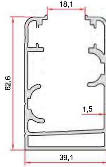
KOD-CODE EP-2621 TEORİK AĞIRLIK THEORETICAL WEIGHT 1,169 Kg/m
