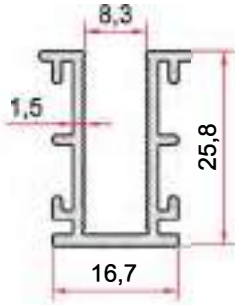
KOD-CODE TEORİK AĞIRLIK THEORETICAL WEIGHT EP-2390 0,345 Kg/m
