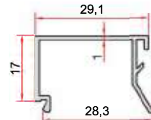
KOD-CODE TEORİK AĞIRLIK EP-0833 THEORETICAL WEIGHT 0,208 Kg/m
