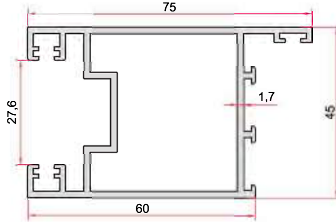
KOD-CODE TEORİK AĞIRLIK THEORETICAL WEIGHT EP-0807 1,280 Kg/m
