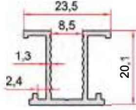
KOD-CODE TEORİK AĞIRLIK THEORETICAL WEIGHT EP-2679 0,256 Kg/m
