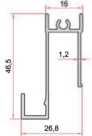
KOD-CODE TEORİK AĞIRLIK THEORETICAL WEIGHT EP-1469 0,413 Kg/m
