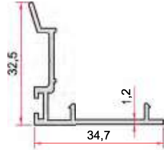
KOD-CODE TEORİK AĞIRLIK THEORETICAL WEIGHT EP-0819 0,283 Kg/m
