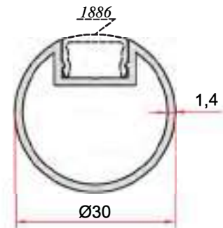
KOD-CODE TEORİK AĞIRLIK THEORETICAL WEIGHT EP-1991 0,391 Kg/m
