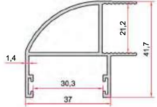
KOD-CODE TEORİK AĞIRLIK EP-2668 THEORETICAL WEIGHT 0,621 Kg/m
