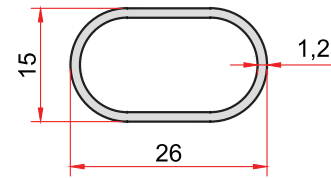
KOD-CODE TEORİK AĞIRLIK THEORETICAL WEIGHT EP-802 0,219 Kg/m
