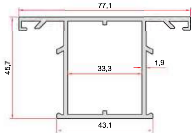
KOD-CODE TEORİK AĞIRLIK EP-0880 THEORETICAL WEIGHT 1,177 Kg/m
