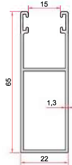
KOD-CODE TEORİK AĞIRLIK THEORETICAL WEIGHT EP-1070 0,623 Kg/m
