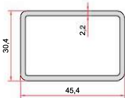
KOD-CODE TEORİK AĞIRLIK THEORETICAL WEIGHT EP-5055 0,823 Kg/m
