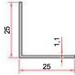
KOD-CODE TEORİK AĞIRLIK EP-0015 THEORETICAL WEIGHT 0,146 Kg/m
