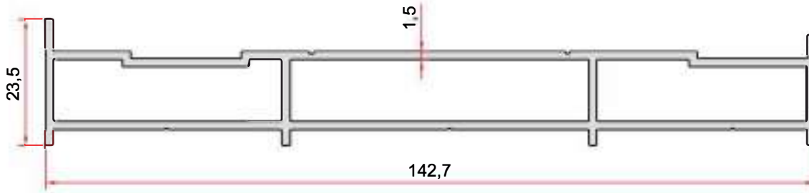
KOD-CODE EP-2672 TEORİK AĞIRLIK THEORETICAL WEIGHT 1,439 Kg/m
