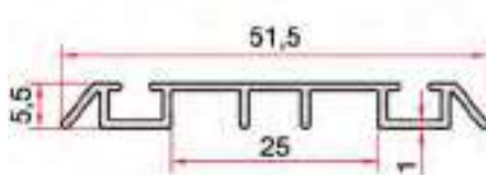
KOD-CODE TEORİK AĞIRLIK THEORETICAL WEIGHT EP-1359 0,240 Kg/m
