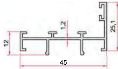
KOD-CODE TEORİK AĞIRLIK THEORETICAL WEIGHT EP-0812 0,383 Kg/m
