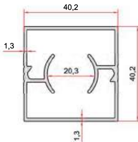
KOD-CODE TEORİK AĞIRLIK THEORETICAL WEIGHT EP-2725 0,748 Kg/m
