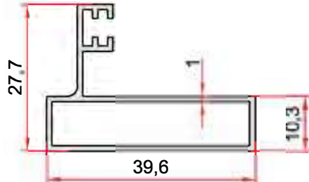
KOD-CODE TEORİK AĞIRLIK THEORETICAL WEIGHT EP-2763 0,356 Kg/m
