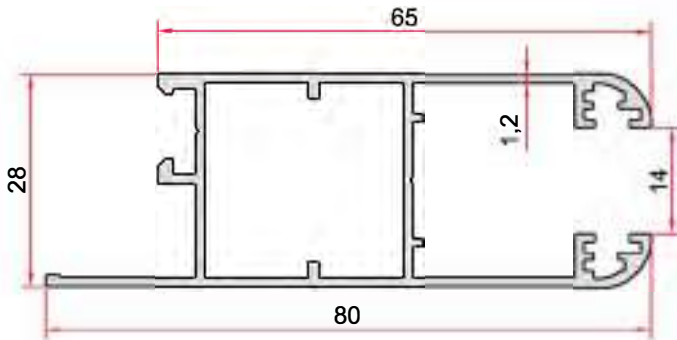
KOD-CODE TEORİK AĞIRLIK THEORETICAL WEIGHT EP-1204 0,810 Kg/m
