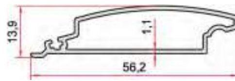
KOD-CODE TEORİK AĞIRLIK THEORETICAL WEIGHT EP-1015 0,365 Kg/m
