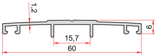
KOD-CODE TEORİK AĞIRLIK EP-1063 THEORETICAL WEIGHT 0,321 Kg/m
