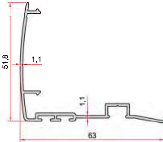
KOD-CODE TEORİK AĞIRLIK THEORETICAL WEIGHT EPKS-4514-11 0,448 Kg/m
