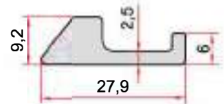
KOD-CODE TEORİK AĞIRLIK THEORETICAL WEIGHT EP-1490 0,362 Kg/m
