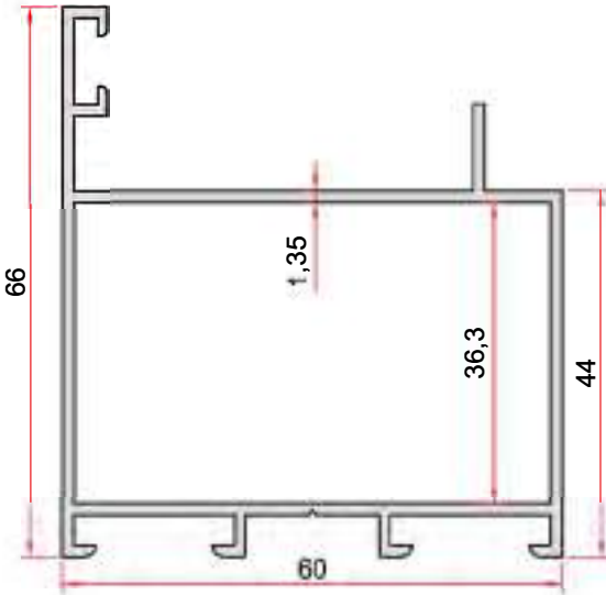
KOD-CODE TEORİK AĞIRLIK THEORETICAL WEIGHT EP-0845 0,967 Kg/m
