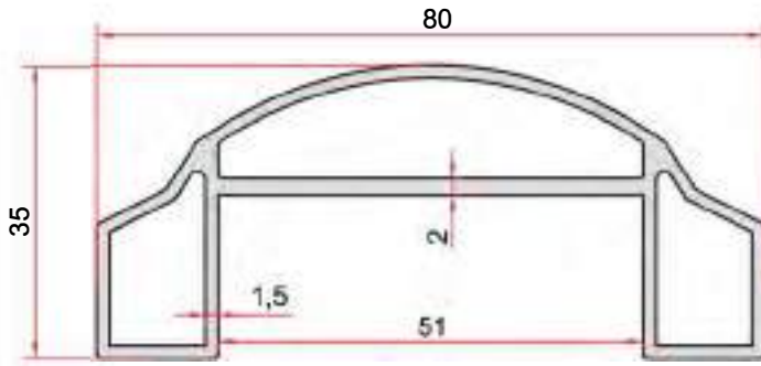
KOD-CODE TEORİK AĞIRLIK THEORETICAL WEIGHT EP-0148 1,075 Kg/m
