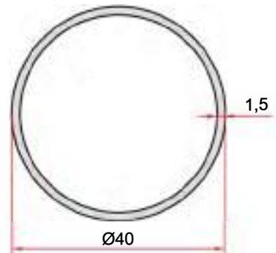
KOD-CODE TEORİK AĞIRLIK THEORETICAL WEIGHT EP-1910 0,489 Kg/m
