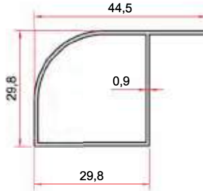
KOD-CODE TEORİK AĞIRLIK THEORETICAL WEIGHT EP-1434 0,297 Kg/m
