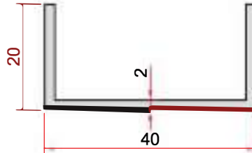
KOD-CODE TEORİK AĞIRLIK THEORETICAL WEIGHT EP-0026 0,410 Kg/m
