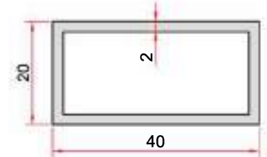
KOD-CODE TEORİK AĞIRLIK THEORETICAL WEIGHT EP-0051 0,605 Kg/m
