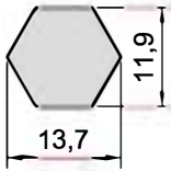
KOD-CODE TEORİK AĞIRLIK THEORETICAL WEIGHT EP-2273 0,332 Kg/m
