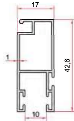
KOD-CODE TEORİK AĞIRLIK THEORETICAL WEIGHT EP-1066 0,389 Kg/m
