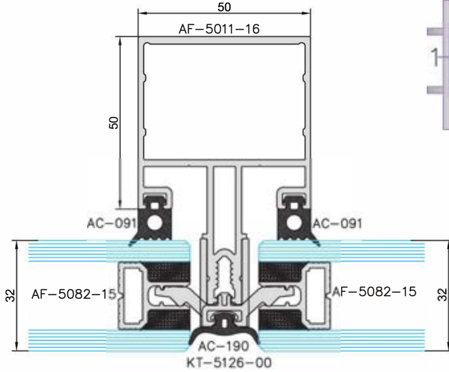
Silikon Cephe Cam Klipsi
