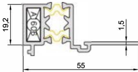
KOD-CODE AF-5075-15 TEORİK AĞIRLIK THEORETICAL WEIGHT 0,786 Kg/m
