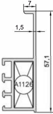
KOD-CODE AF-5069-15 TEORİK AĞIRLIK THEORETICAL WEIGHT 0,575 Kg/m
