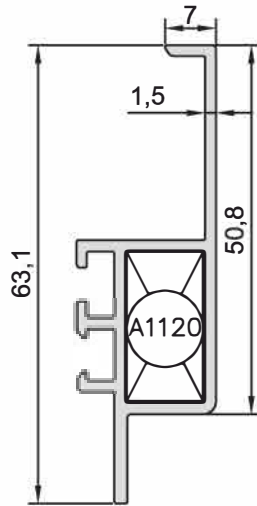
KOD-CODE AF-5070-15 TEORİK AĞIRLIK THEORETICAL WEIGHT 0,561 Kg/m
