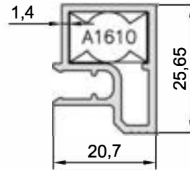
KOD-CODE AF-5076-16 TEORİK AĞIRLIK THEORETICAL WEIGHT 0,386 Kg/m
