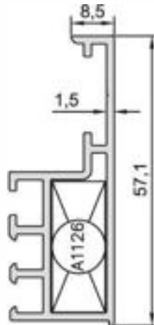
KOD-CODE AF-5073-15 TEORİK AĞIRLIK THEORETICAL WEIGHT 0,647 Kg/m
