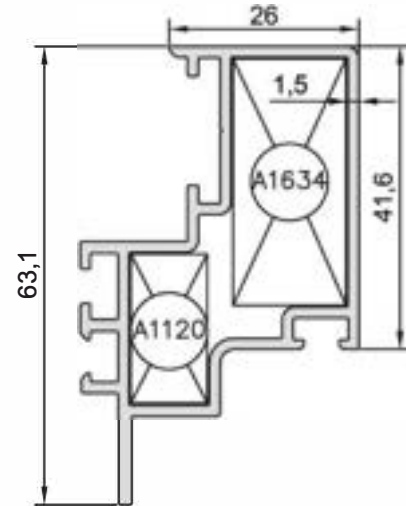
KOD-CODE AF-5071-15 TEORİK AĞIRLIK THEORETICAL WEIGHT 0,867 Kg/m
