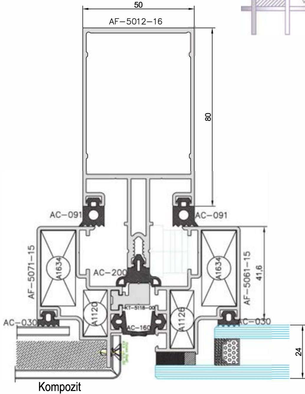
Silikon Cephe Kasetli Kompozit Detayı
