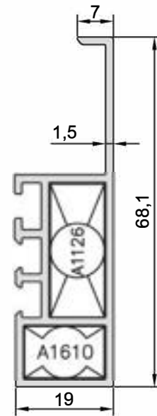
KOD-CODE AF-5074-15 TEORİK AĞIRLIK THEORETICAL WEIGHT 0,735 Kg/m
